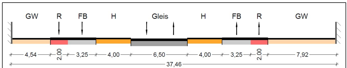
Abbildung 11: Hauptvariante 2, TS, geplanter Querschnitt auf Höhe Haus Nr. 15 / Haltestelle Innere Klosterstraße (Angaben in Meter), Quelle: Voruntersuchung
