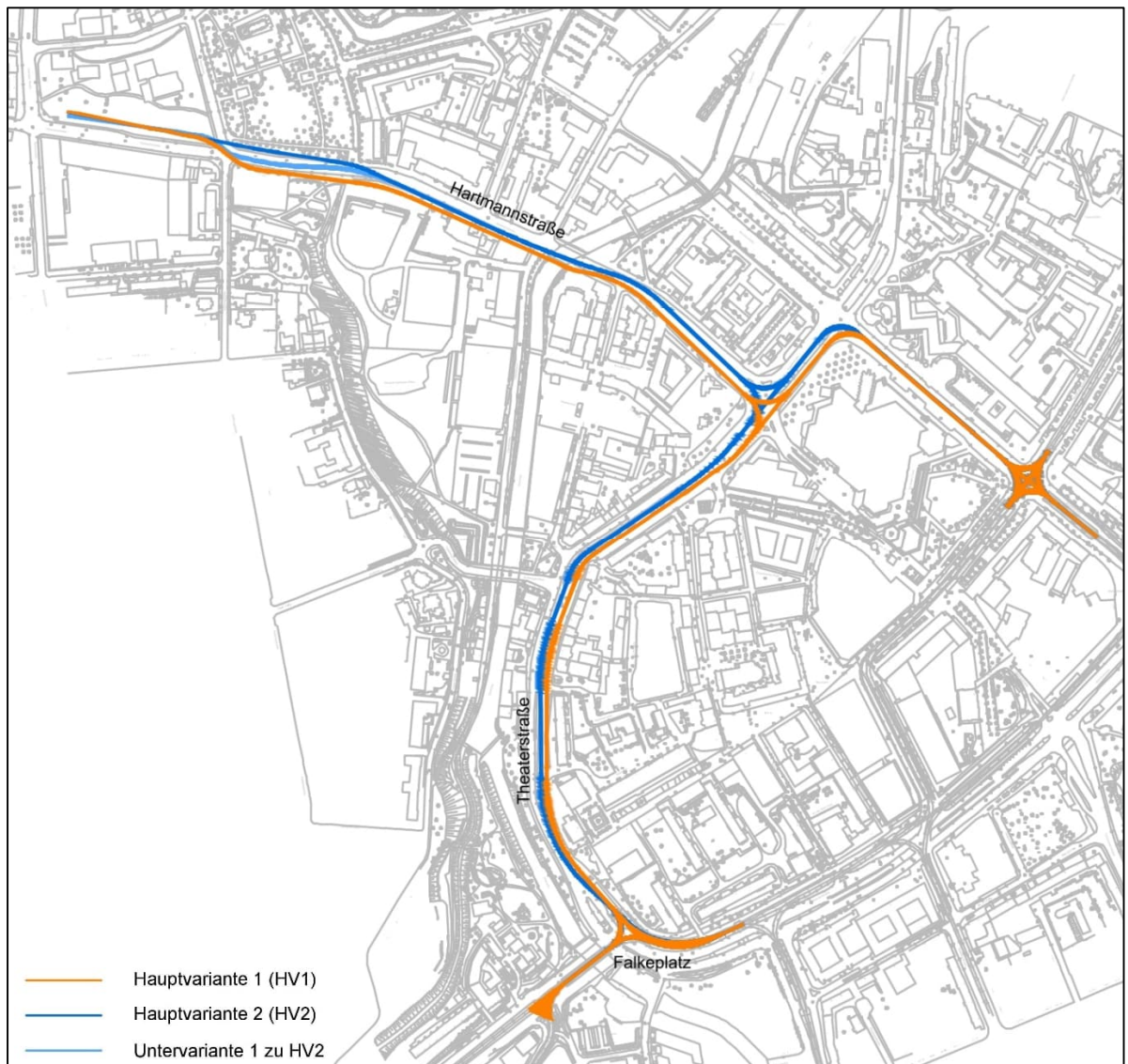
Abbildung 6: Übersichtslageplan der untersuchten Varianten (Darstellung der Gleistrassen)
