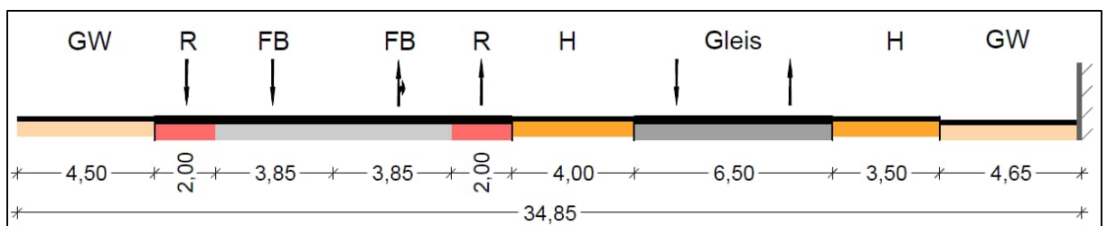
Abbildung 9: Hauptvariante 1, HS, geplanter Querschnitt Haltestelle Theaterstraße (Angabe in Meter), Quelle: Voruntersuchung
