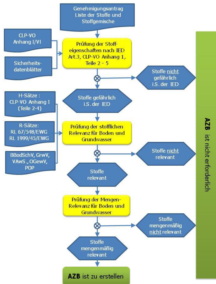
Abbildung 5: Fließschema zur Relevanzprüfung von Stoffen und Gemischen aus Ad-hoc AG – Arbeitshilfe zum AZB [7]
