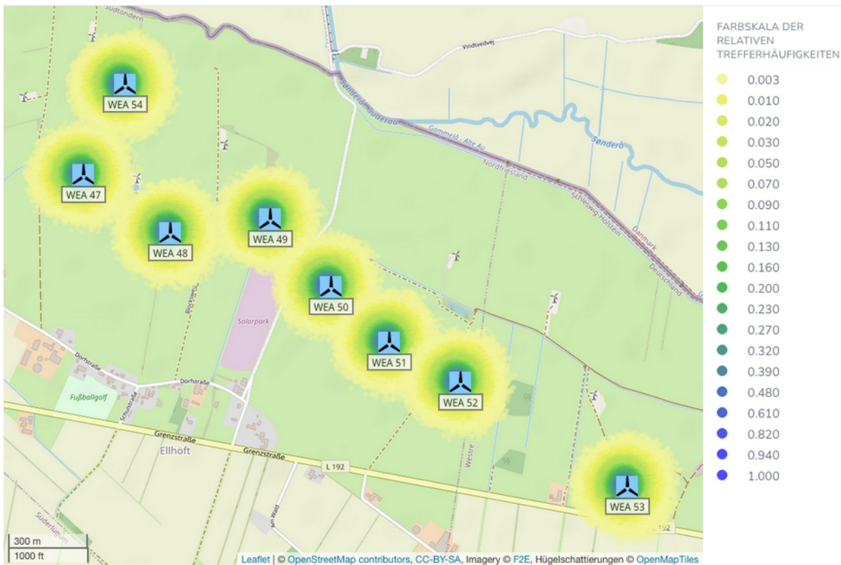
Abbildung A.1.1: Trefferhäufigkeiten von Eisstücken pro Rasterfläche (16m 2 ) und Jahr in der Umgebung der WEA 47 - 54 am Standort Neubau 8 WEA, Ellhöft/Westre (Karte /1.4/).
