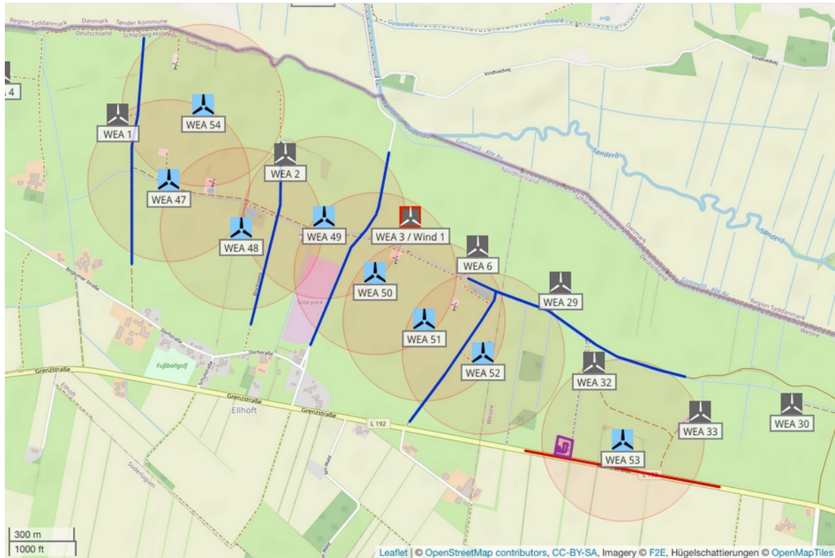
Abbildung 4.3.1: Potentielle Gefährdungsbereiche der WEA und Schutzobjekte am Standort Neubau 8 WEA, Ellhöft/Westre (Karte 1/1.4/).
