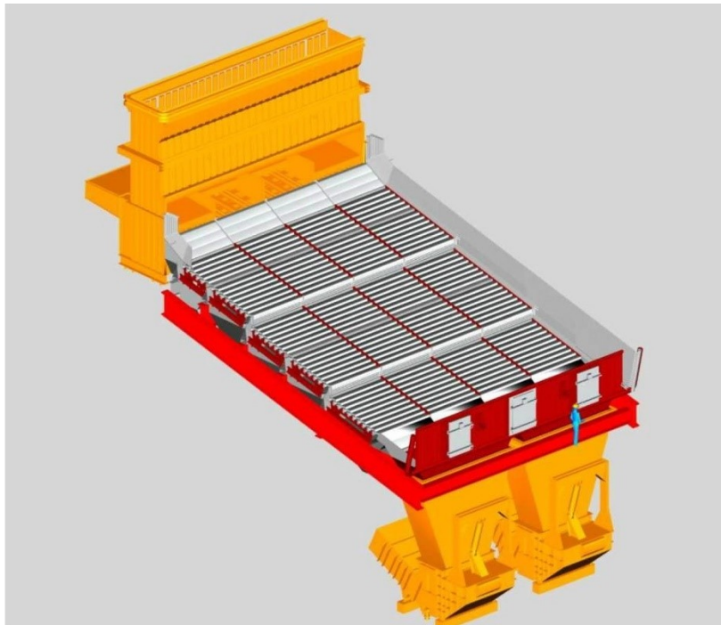
Abbildung 8 Beispielhafte Darstellung des Rostes (Quelle: SBEng)
