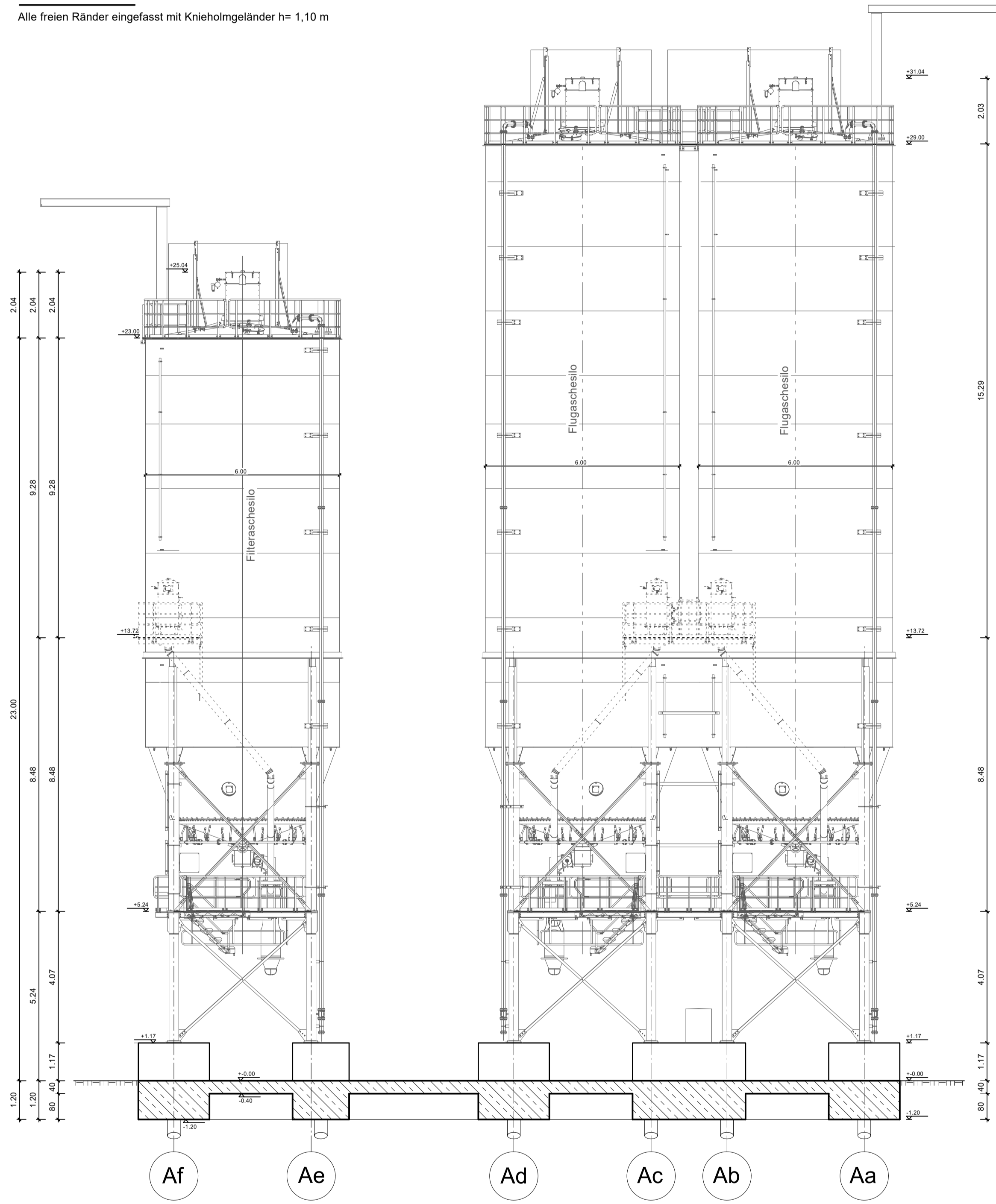
Schnitt C-C Alle freien Ränder eingefasst mit Knieholmgeländer h= 1,10 m
