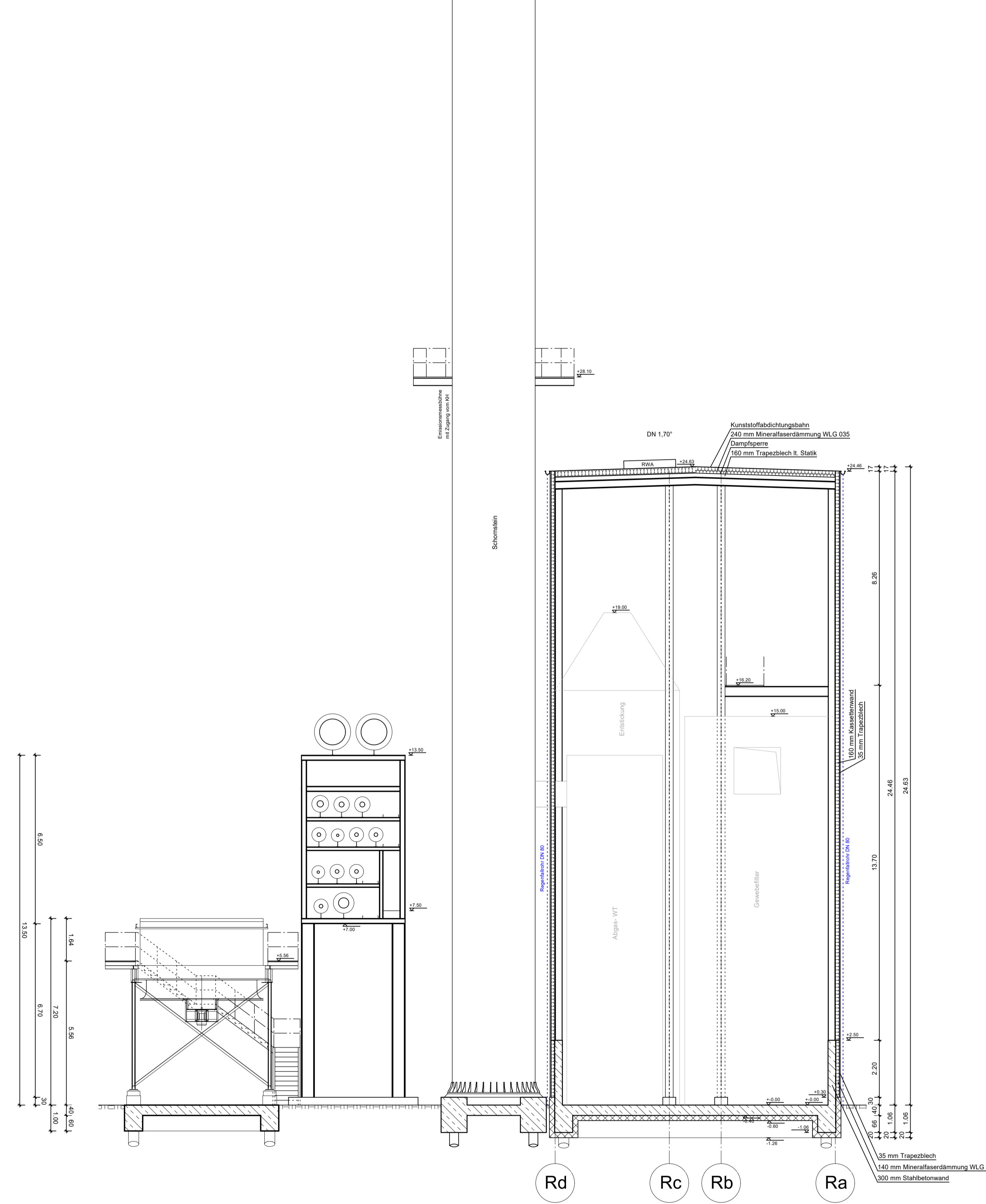
Schnitt D-D Aschenlos und Treppenturm nicht mit dargestellt Alle freien Ränder eingefasst mit Knieholmgeländer h= 1,10 m
