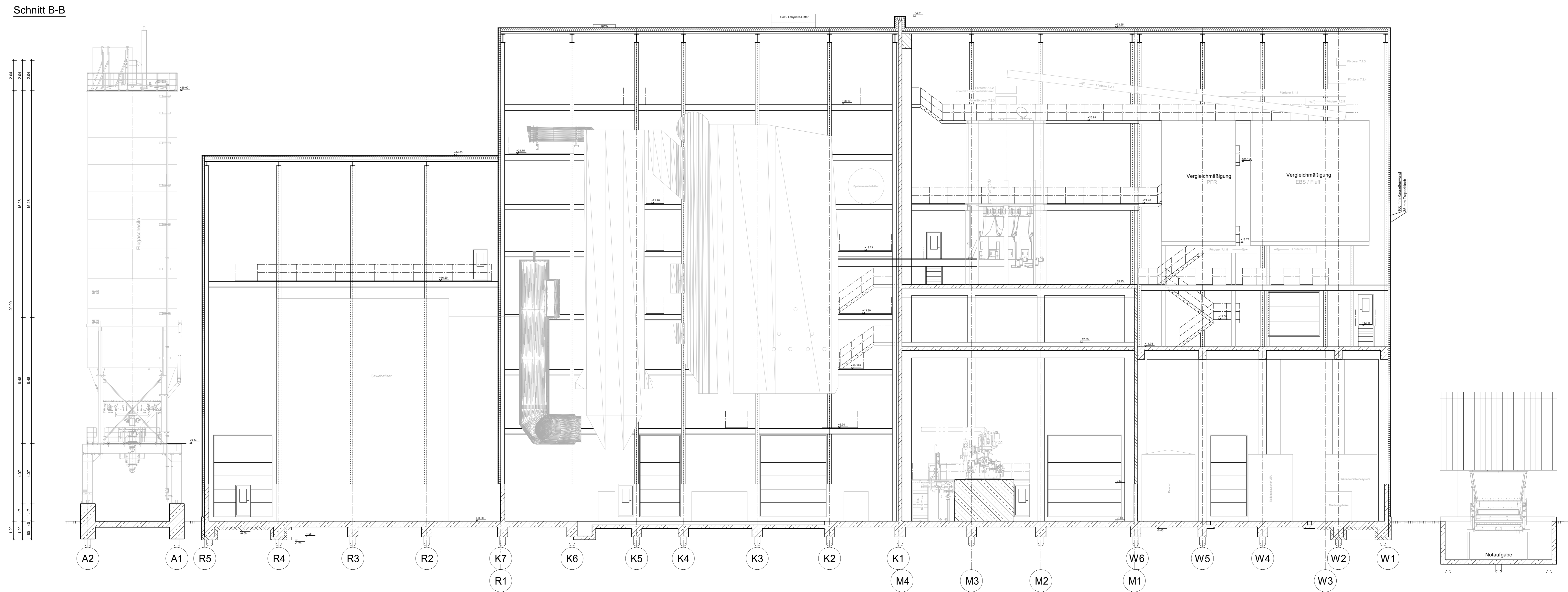
Schnitt B-B
