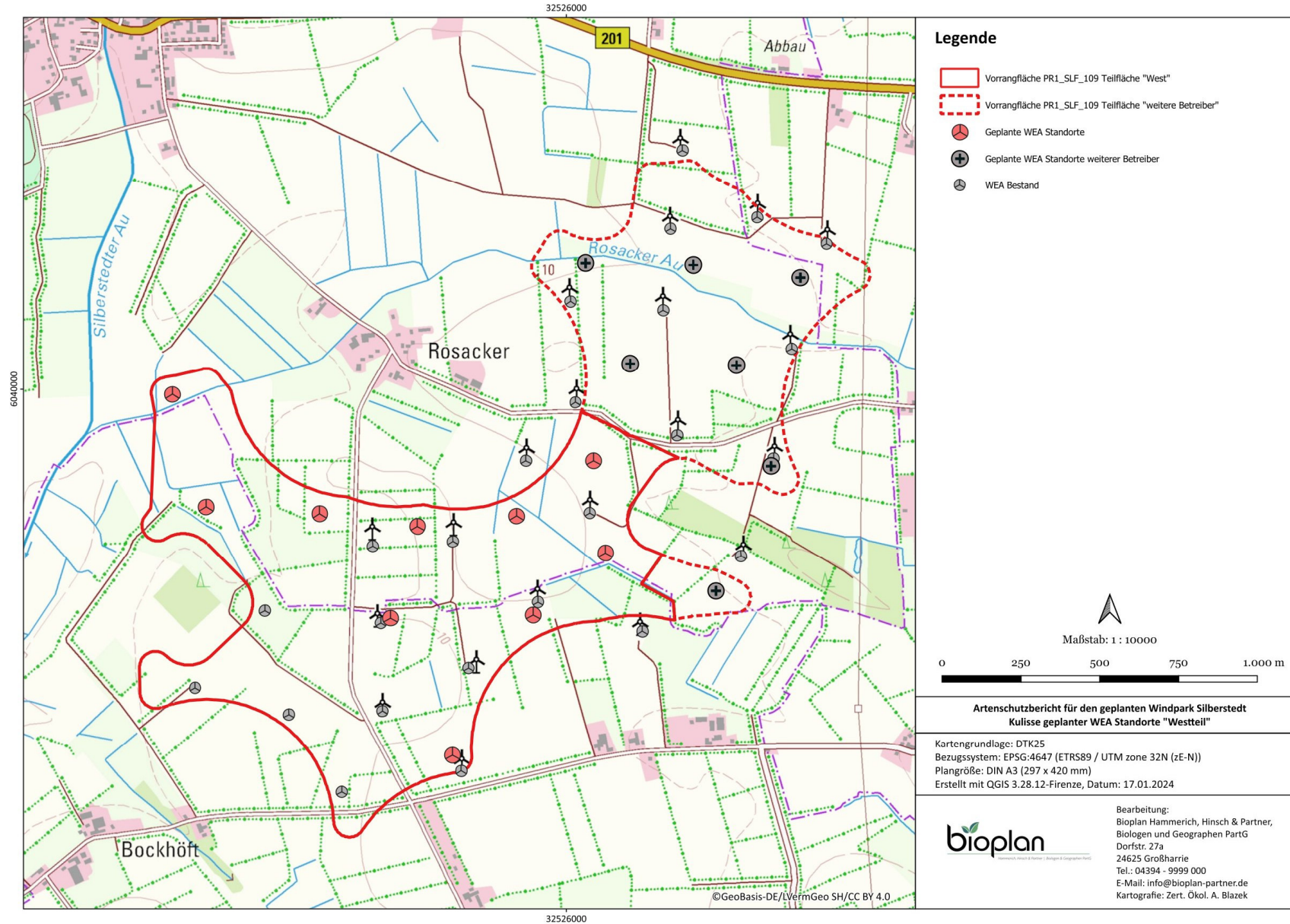
Abbildung 2: Kulisse geplanter WEA Standorte Teilfläche West (eigene Darstellung)
