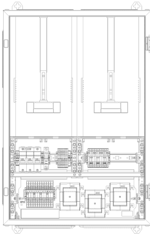
Abb. 2: Zählerbox
