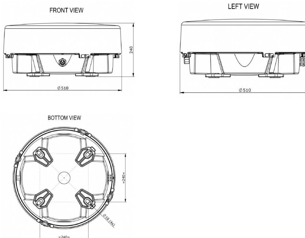
Abbildung 5-1: Gefahrenfeuer – Abmessungen
