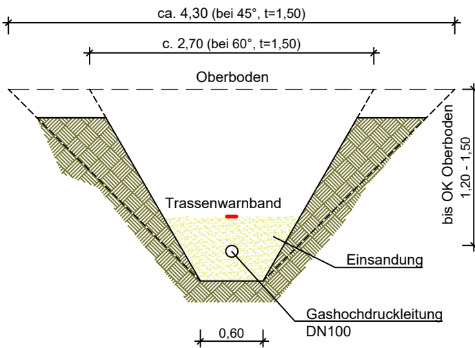
Abbildung 2: Grabenquerschnitt DN 100 - geböschst (M. 1:50)
