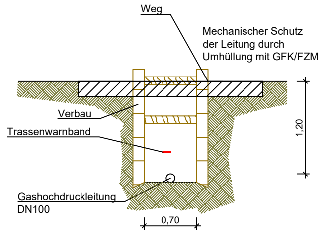
Abbildung 3: Grabenquerschnitt DN 100 - verbaut in Wegeflächen (M. 1:50)
