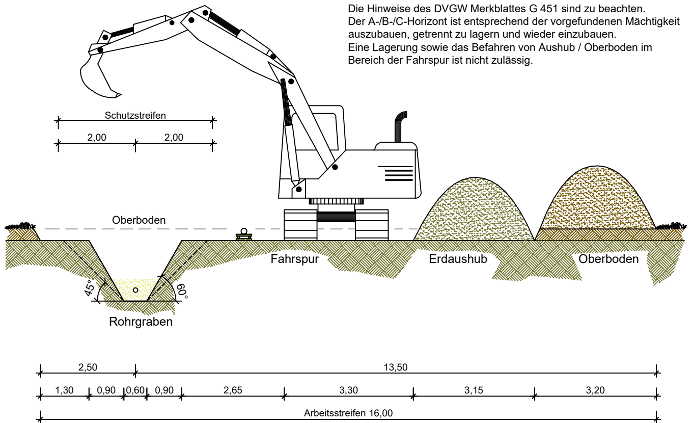
Abbildung 1: Arbeitsstreifen DN 100, freie Verlegestrecke (M. 1:100)
