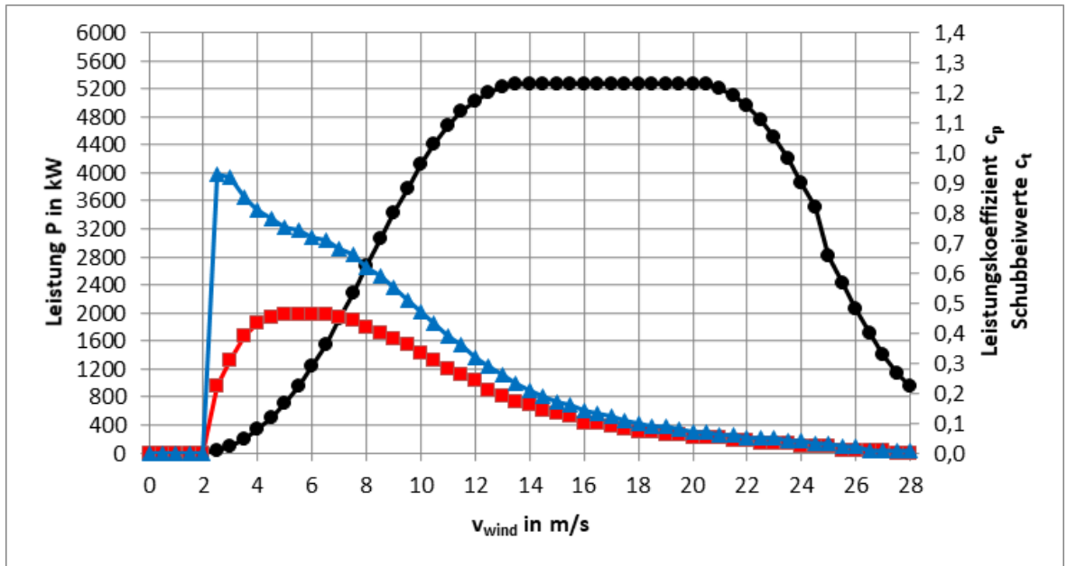
Abb. 2: Leistungs-, c_p - und c_t -Kennlinien E-160 EP5 E3 / 5560 kW Betriebsmodus NR II s
