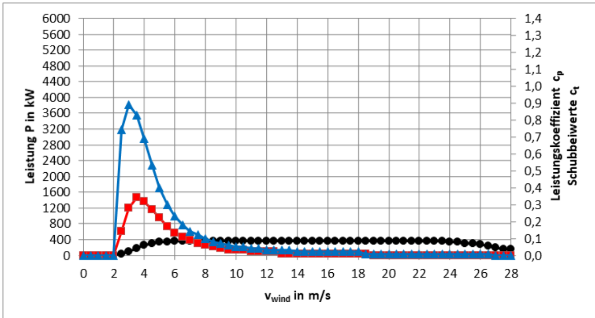
Abb. 9: Leistungs-, c_p - und c_t -Kennlinien E-160 EP5 E3 / 5560 kW Betriebsmodus NR IX s
