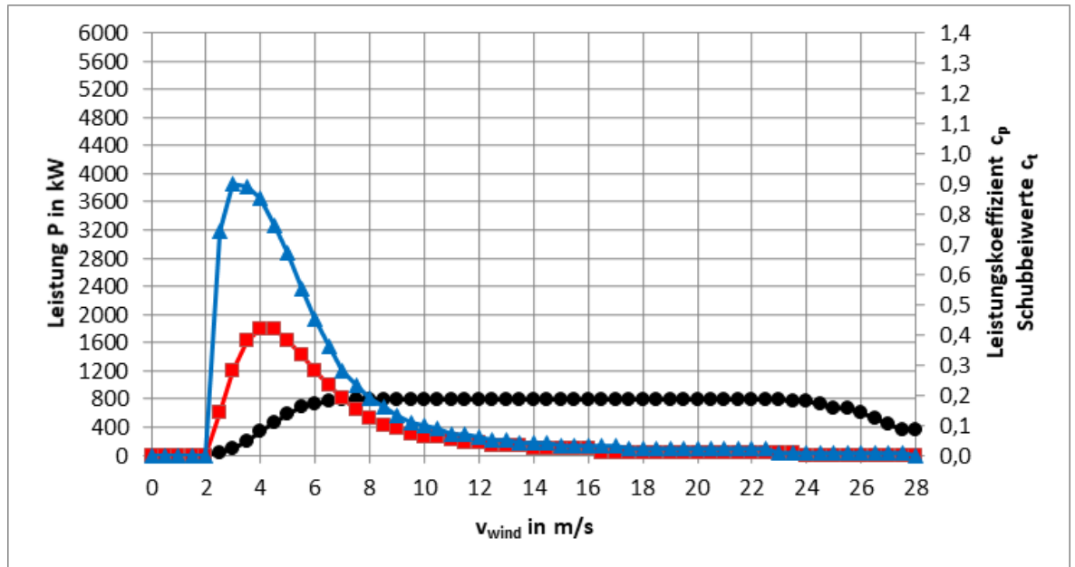
Abb. 8: Leistungs-, c_p - und c_t -Kennlinien E-160 EP5 E3 / 5560 kW Betriebsmodus NR VIII s
