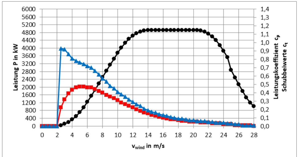
Abb. 4: Leistungs-, c_p - und c_t -Kennlinien E-160 EP5 E3 / 5560 kW Betriebsmodus NR IV s
