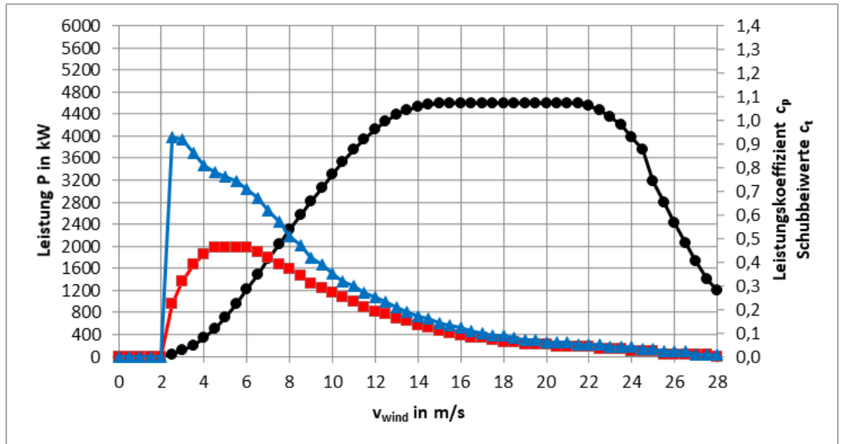
Abb. 6: Leistungs-, c_p - und c_t -Kennlinien E-160 EP5 E3 / 5560 kW Betriebsmodus NR VI s
