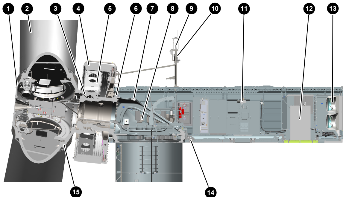
Abb. 1: Gondelschnitt
