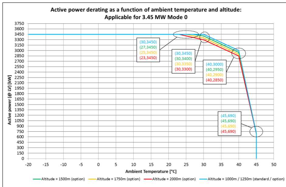
Abbildung 10-1: Temperatur- und höhenbedingter Teillastbetrieb im 3,45-MW-Modus 0
