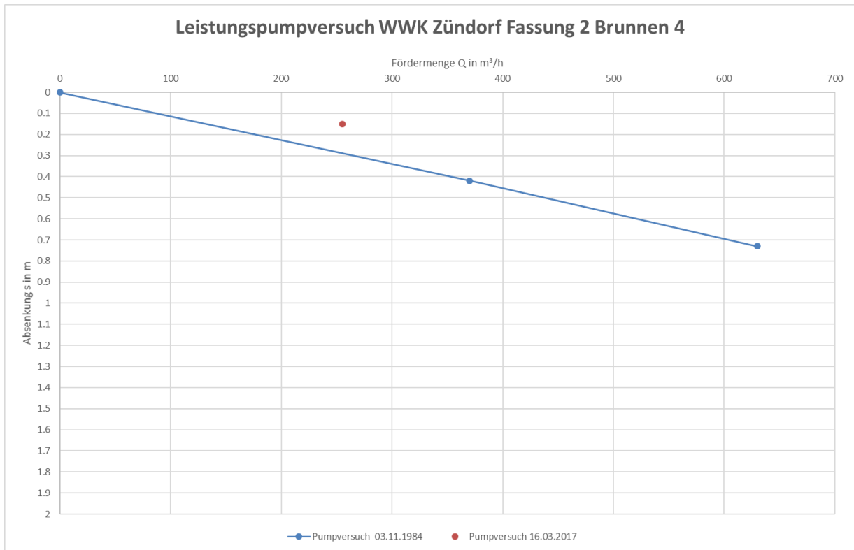
Leistungscharakteristik Brunnen ZD 2.4
