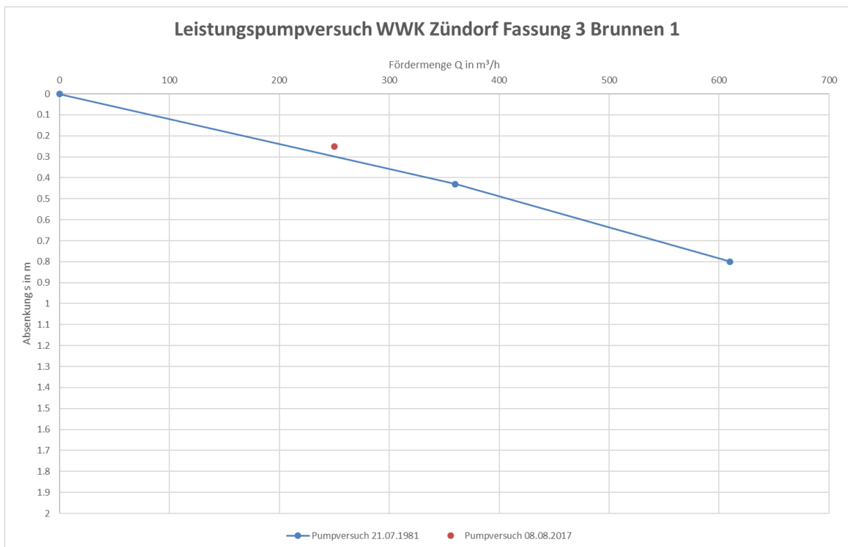
Leistungscharakteristik Brunnen ZD 3.1
