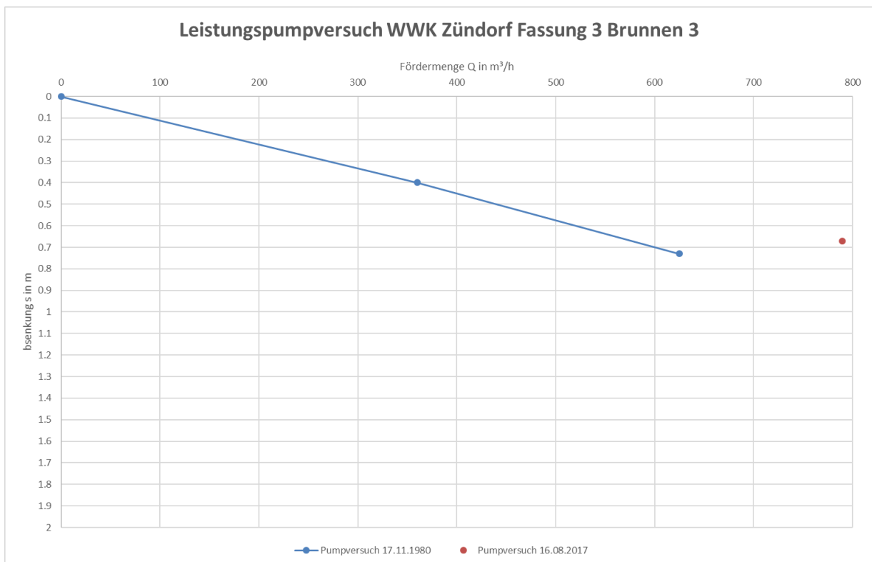
Leistungscharakteristik Brunnen ZD 3.3
