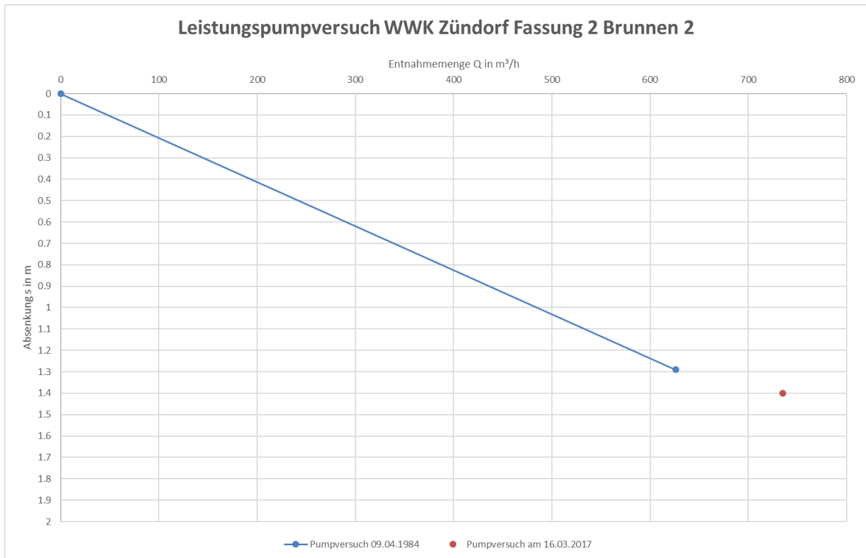
Leistungscharakteristik Brunnen ZD 2.2
