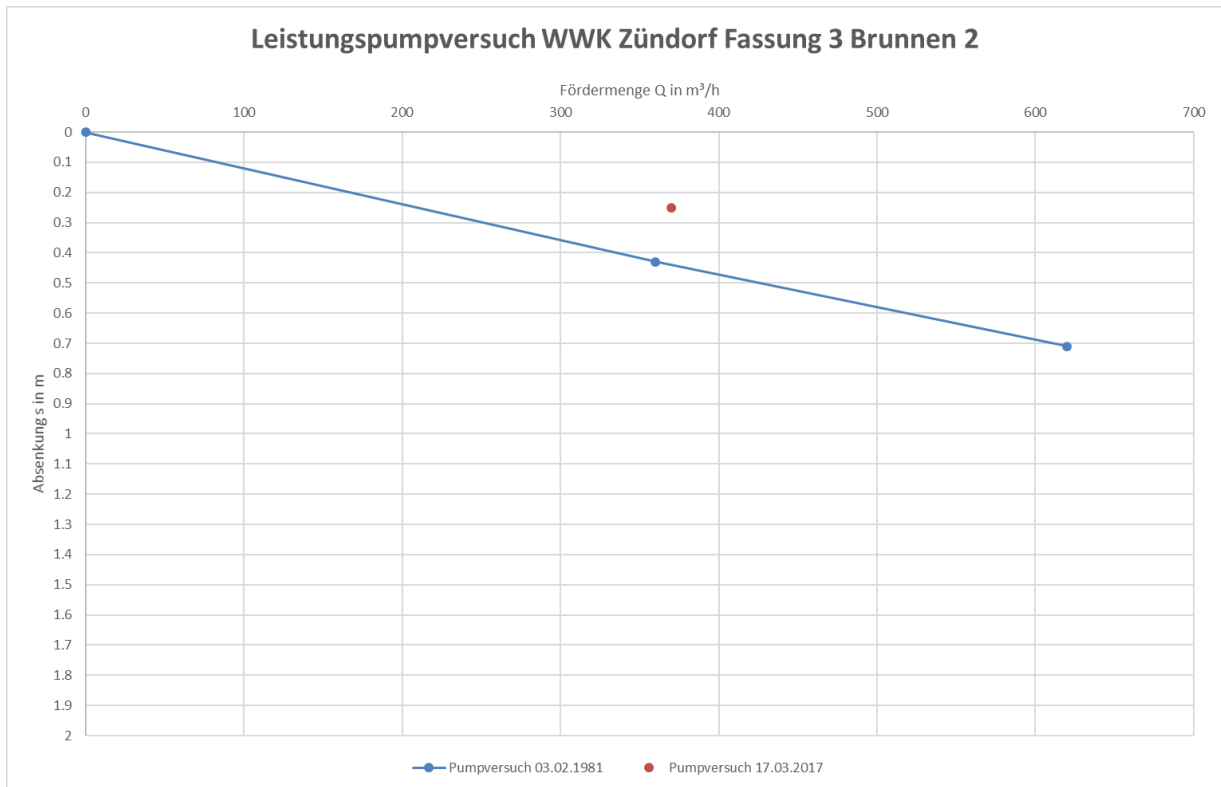
Leistungscharakteristik Brunnen ZD 3.2
