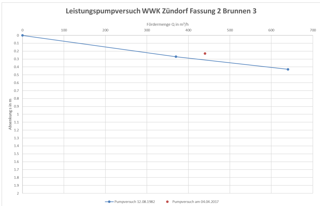
Leistungscharakteristik Brunnen ZD 2.3
