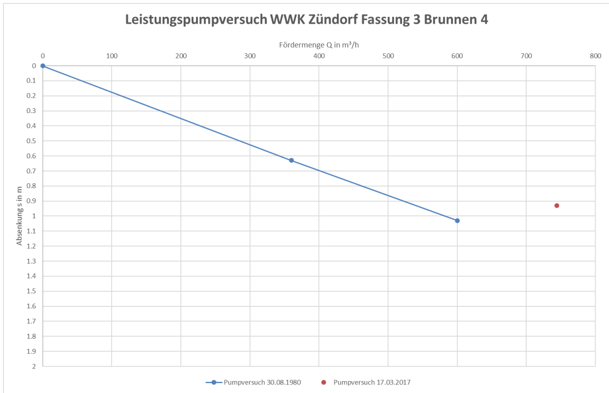
Leistungscharakteristik Brunnen ZD 3.4
