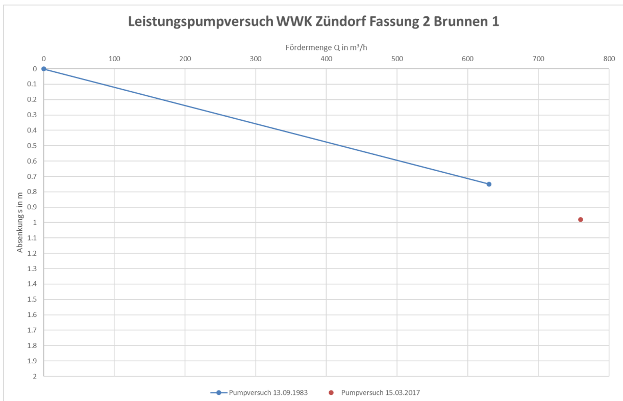
Leistungscharakteristik Brunnen ZD 2.1
