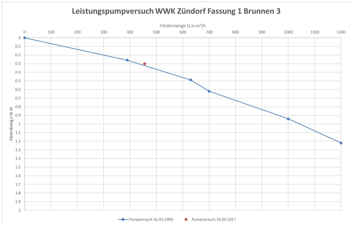
Leistungscharakteristik Brunnen ZD 1.3
