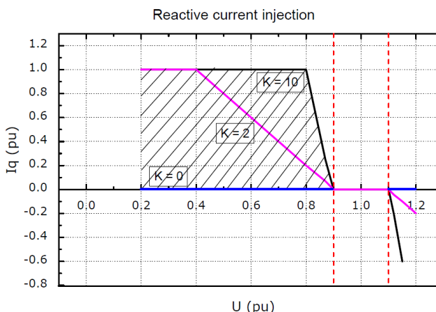
Abbildung 10-2: Blindstromeinspeisung
