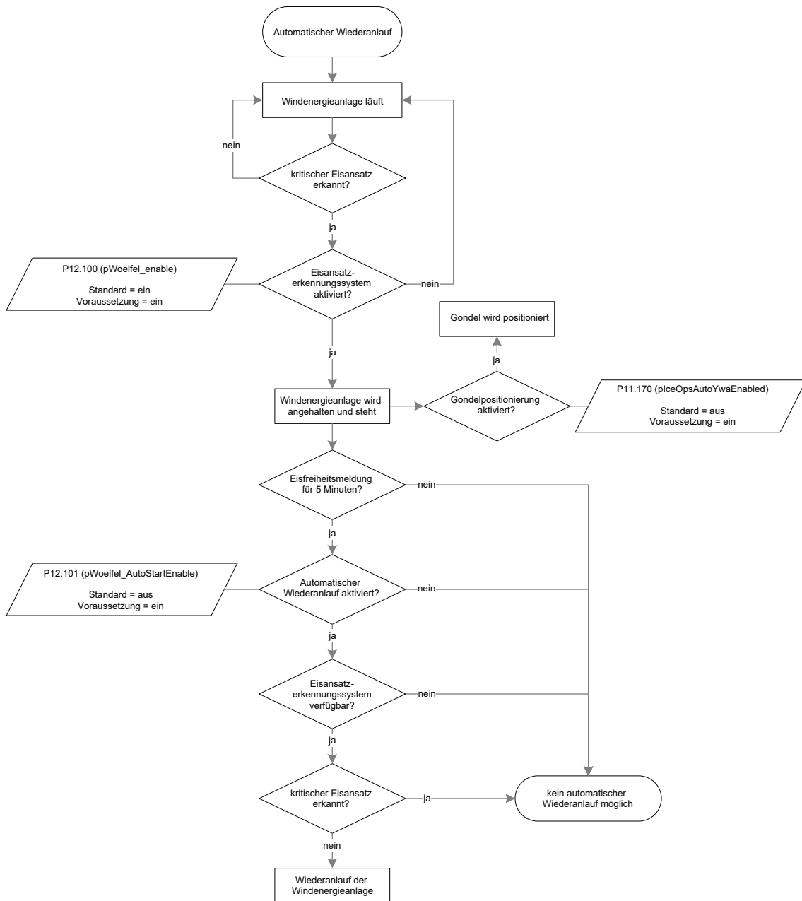
Abb. 6: Automatischer Wiederanlauf
