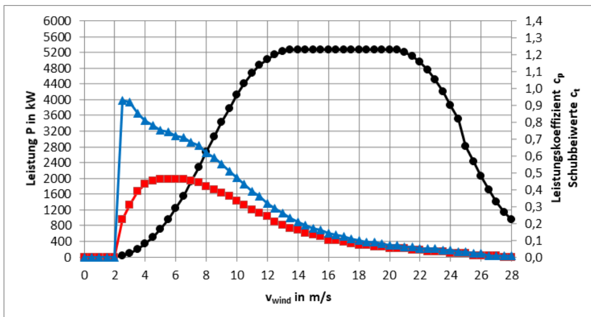
Abb. 2: Leistungs-, c_p - und c_t -Kennlinien E-160 EP5 E3 R1 / 5560 kW Betriebsmodus NR II s
