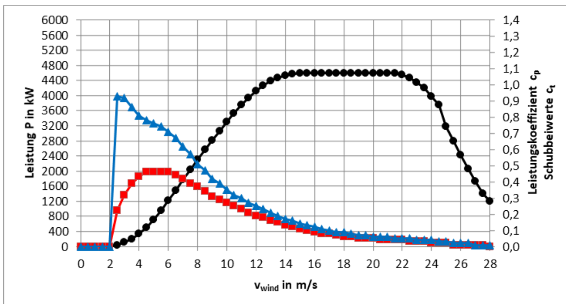
Abb. 6: Leistungs-, c_p - und c_t -Kennlinien E-160 EP5 E3 R1 / 5560 kW Betriebsmodus NR VI s
