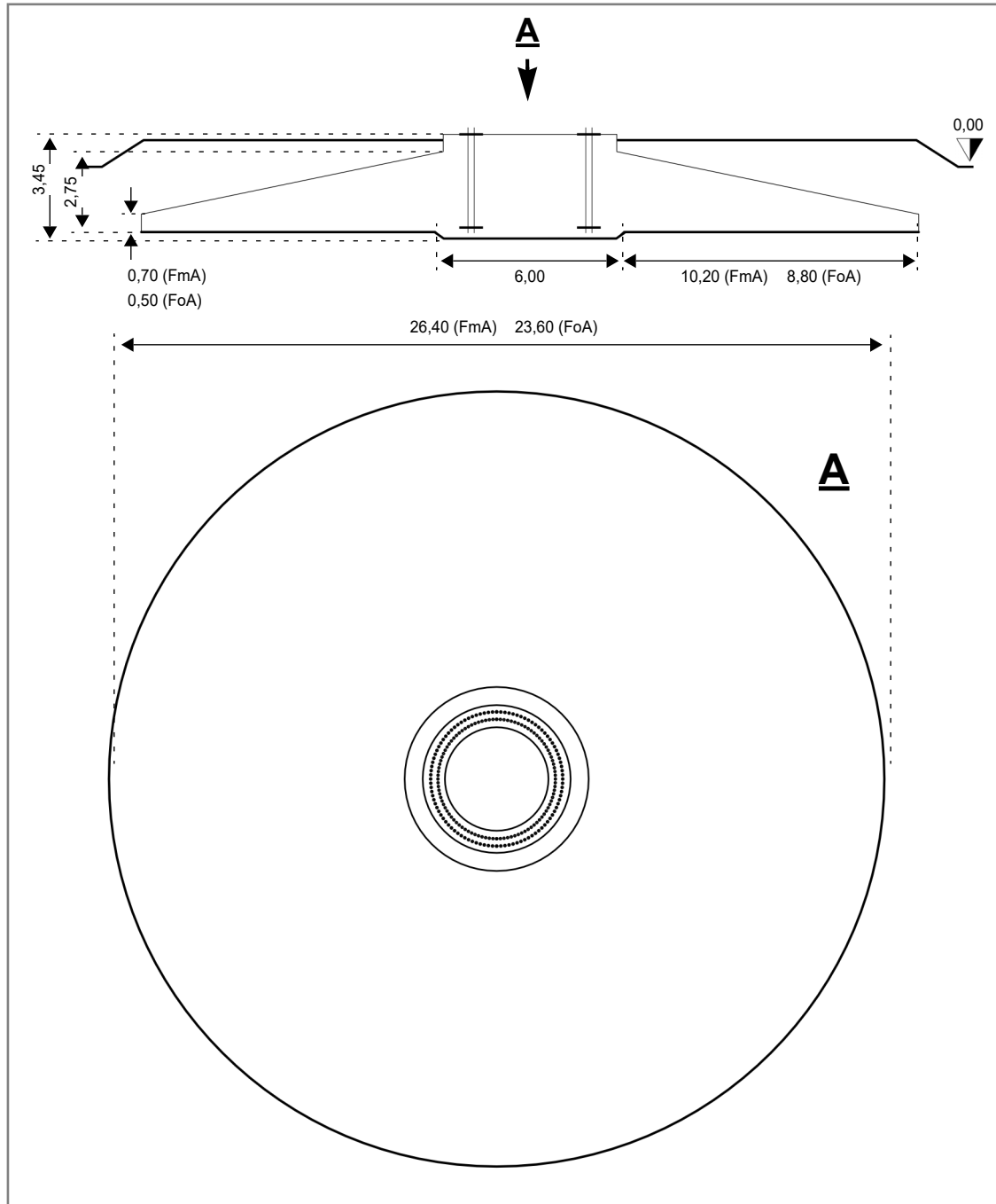
Abb. 1: Darstellung eines Typenfundaments für eine N149/5.X mit 125 m Nabhöhe (alle Angaben in Metern, nicht maßstabgerecht)
