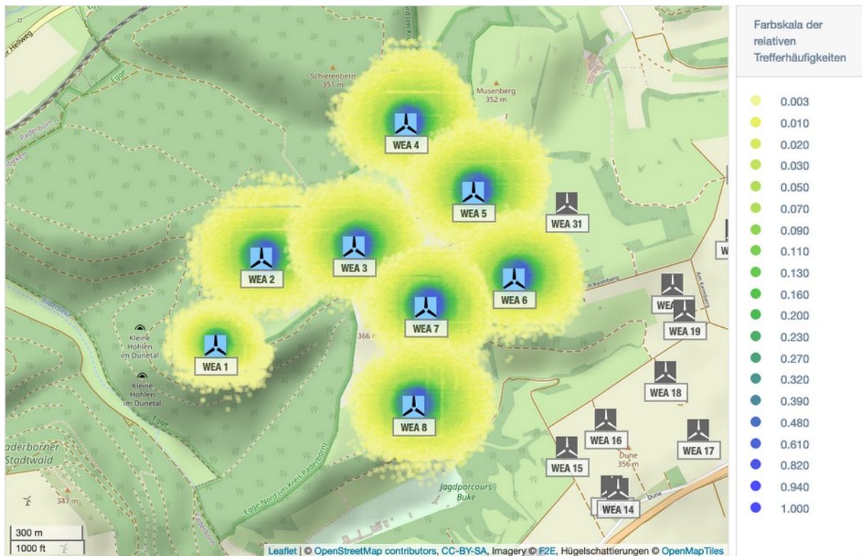
Abbildung A.1.1: Trefferhäufigkeiten von Eisstücken pro Rasterfläche (16m 2 ) und Jahr in der Umgebung der WEA 1 - 8 am Standort Keimberg (Karte /1.4/).
