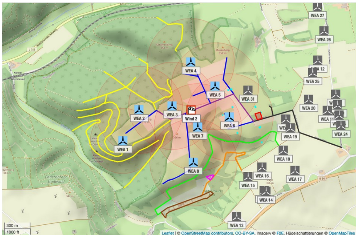
Abbildung 4.3.1: Potentielle Gefährdungsbereiche der WEA 1 - 8 und Schutzobjekte am Standort Keimberg (Karte /1.4/).
