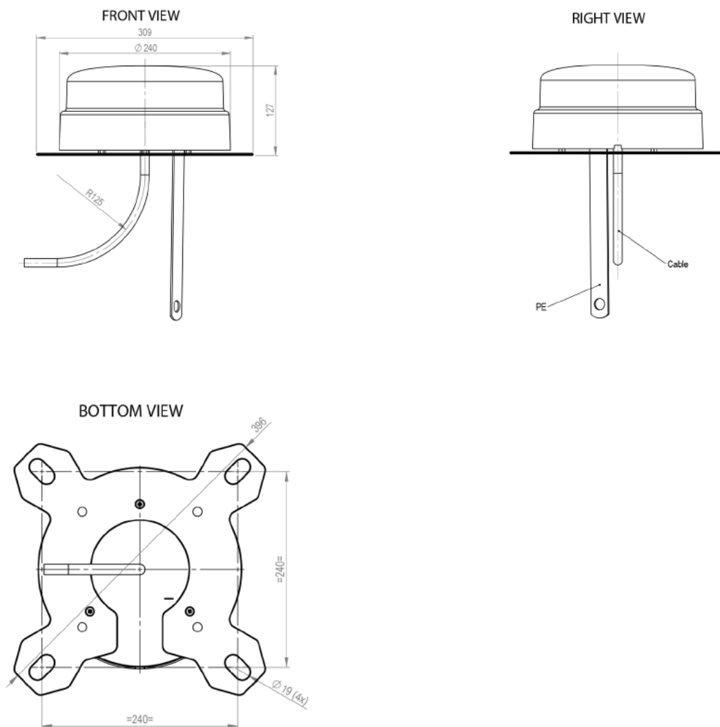
Abbildung 5: Gefahrenfeuer – Maße
