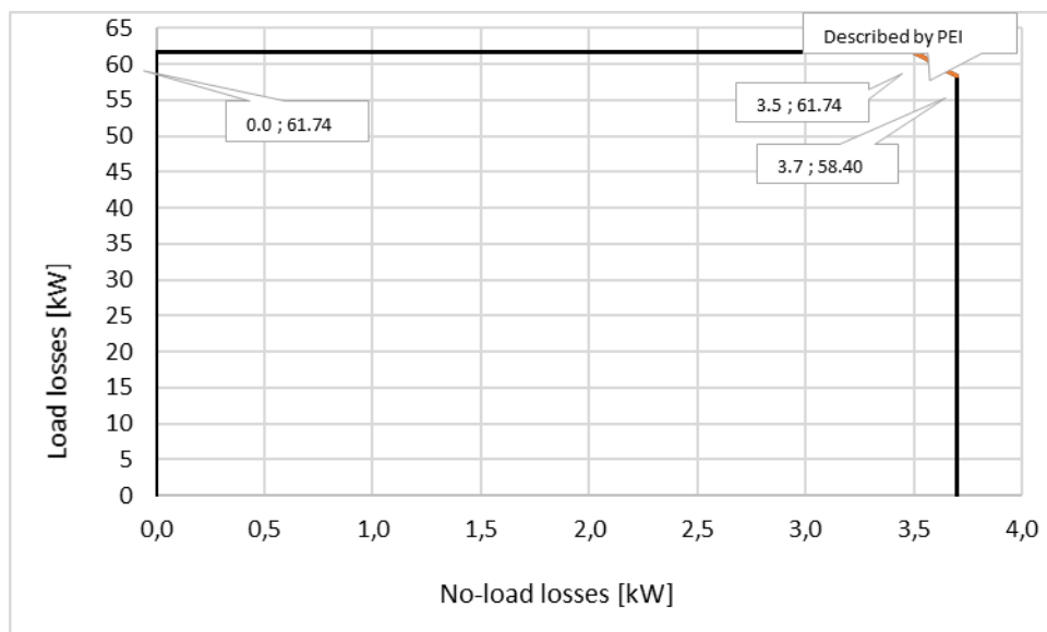
Abbildung 4-1- Transformatorverluste – zulässiger Bereich
