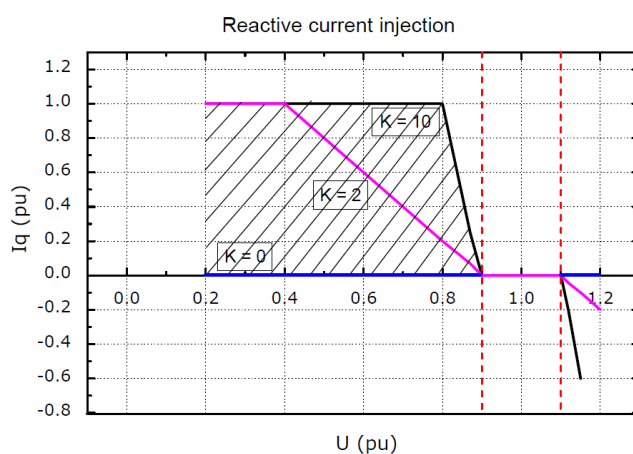
Abbildung 10-2: Blindstromeinspeisung
