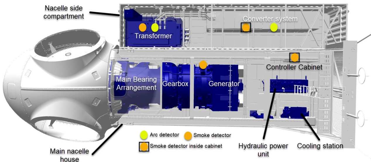
Abbildung 8.1: Prinzipzeichnung des Maschinenhauses von EnVentus™. Der endgültige Einbauort der Sensoren kann angepasst werden.
