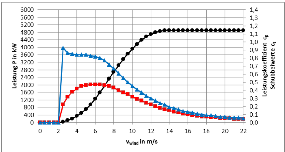
Abb. 3: Leistungs-, c_p - und c_t -Kennlinien E-160 EP5 E2 / 5500 kW Betriebsmodus 104,5 dB
