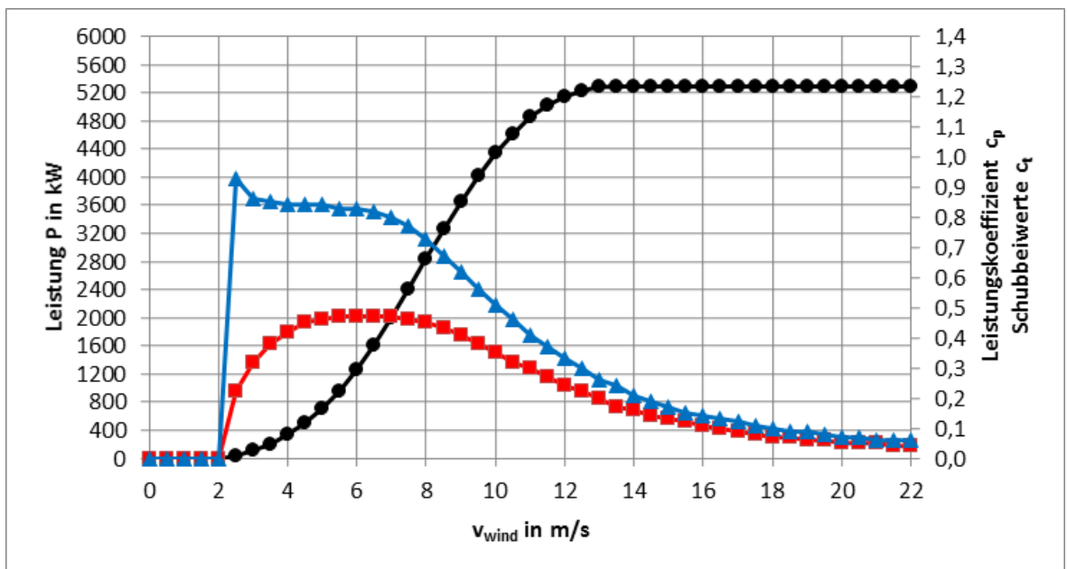
Abb. 1: Leistungs-, c p - und c t -Kennlinien E-160 EP5 E2 / 5500 kW Betriebsmodus 106,0 dB
