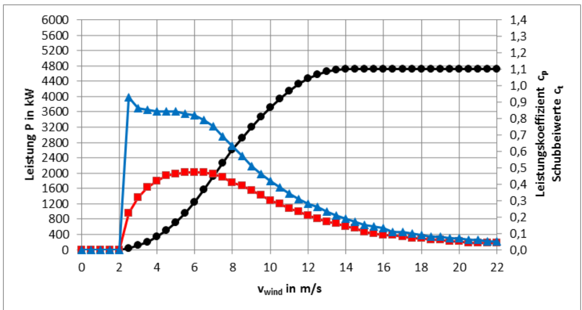
Abb. 4: Leistungs-, c p - und c t -Kennlinien E-160 EP5 E2 / 5500 kW Betriebsmodus 103,7 dB
