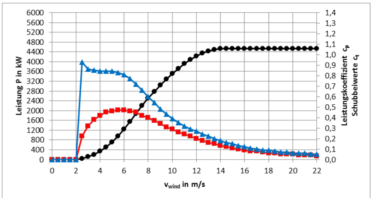
Abb. 5: Leistungs-, c p - und c t -Kennlinien E-160 EP5 E2 / 5500 kW Betriebsmodus 102,9 dB
