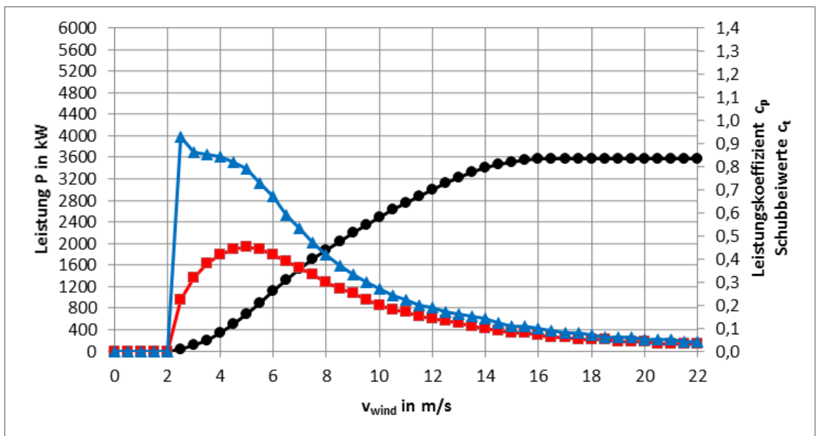
Abb. 8: Leistungs-, c p - und c t -Kennlinien E-160 EP5 E2 / 5500 kW Betriebsmodus 98,0 dB
