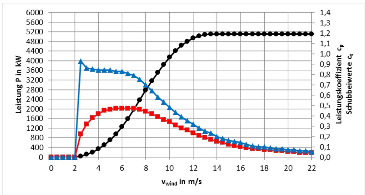
Abb. 2: Leistungs-, c_p - und c_t -Kennlinien E-160 EP5 E2 / 5500 kW Betriebsmodus 105,2 dB
