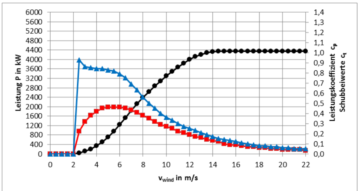
Abb. 6: Leistungs-, c p - und c t -Kennlinien E-160 EP5 E2 / 5500 kW Betriebsmodus 102,0 dB
