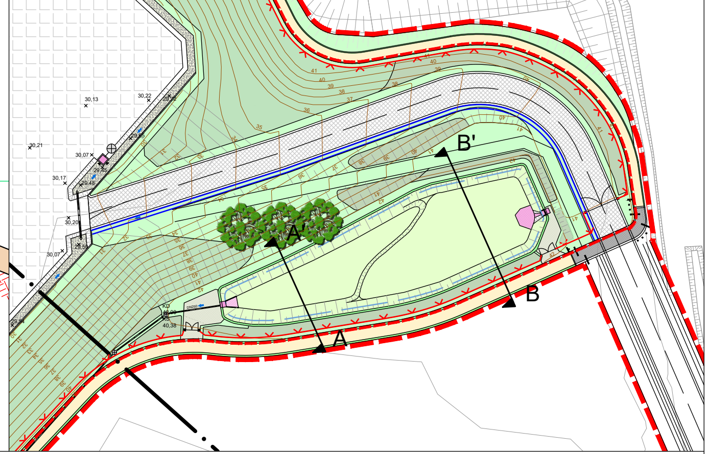
Lage der Schnitte M1:1.000
