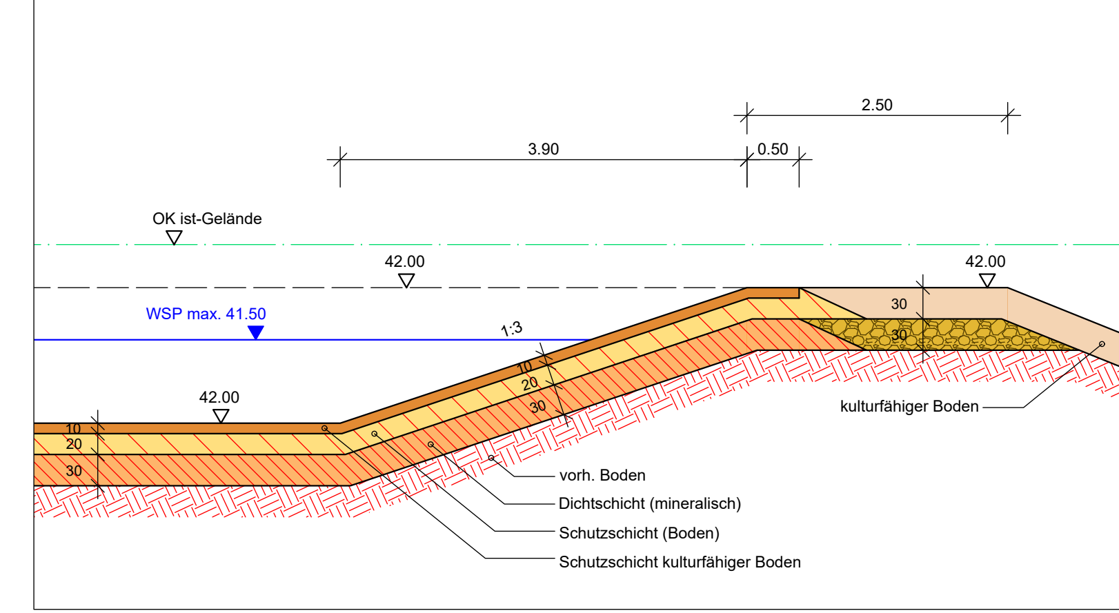
Regelaufbau Beckensohle M1:50
