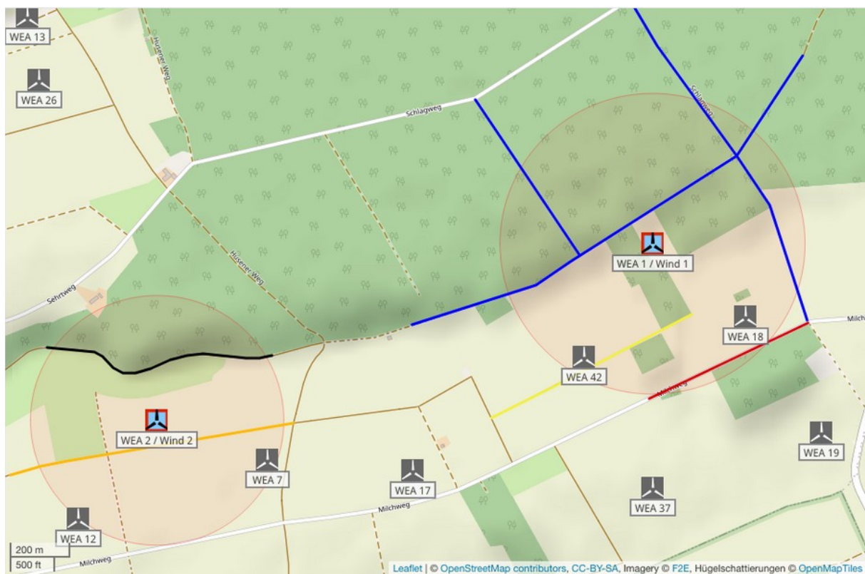
Abbildung 4.3.1: Potentielle Gefährdungsbereiche der WEA und Schutzobjekte am Standort Borchten-Etteln (Karte /1.4/).
