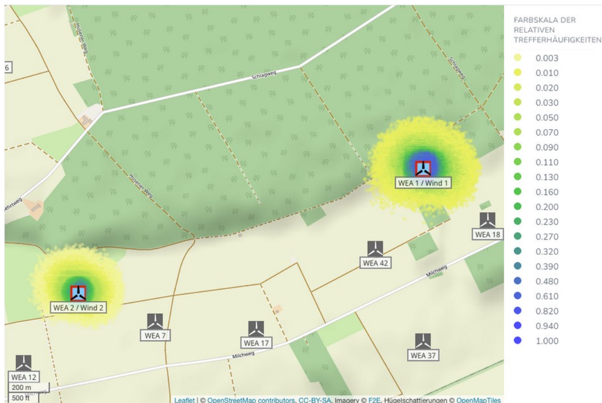
Abbildung A.1.1: Trefferhäufigkeiten von Eisstücken pro Rasterfläche (16m 2 ) und Jahr in der Umgebung der WEA 1 und 2 am Standort Borchten-Etteln (Karte 1/4/).
