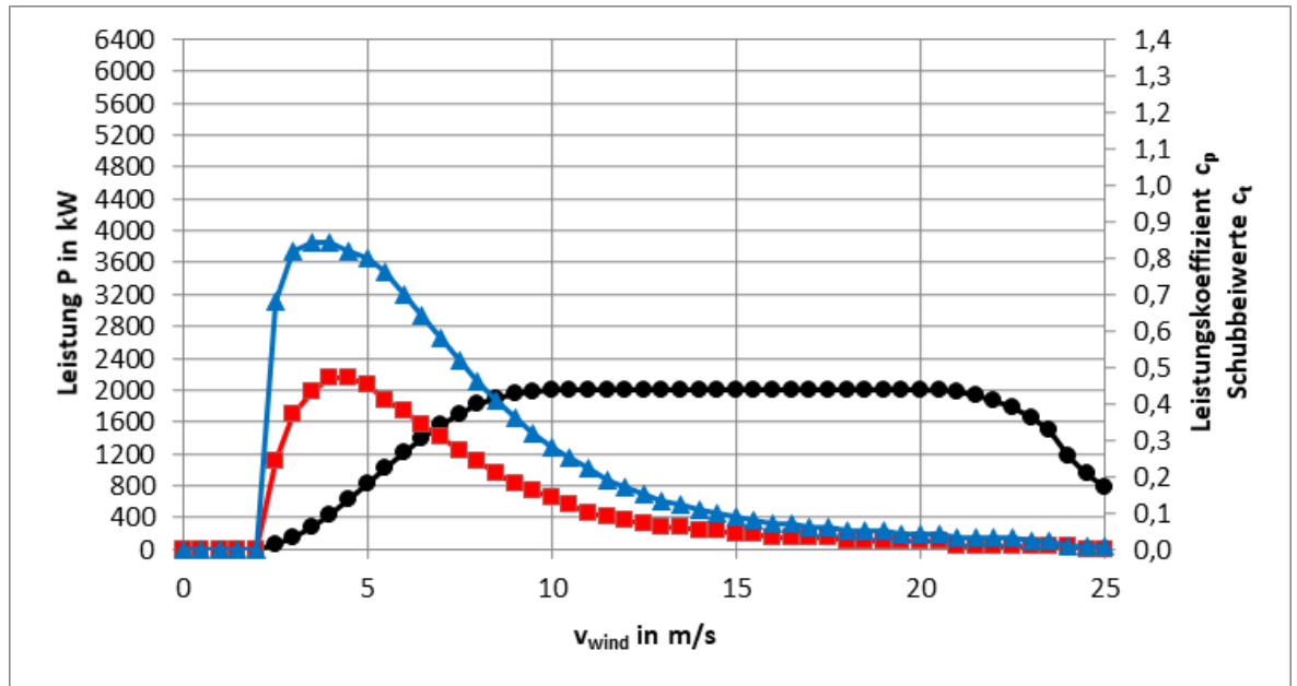
Abb. 1: Leistungs-, c_p - und c_t -Kennlinien E-175 EP5 / 6000 kW Betriebsmodus OM-NR-08-0
