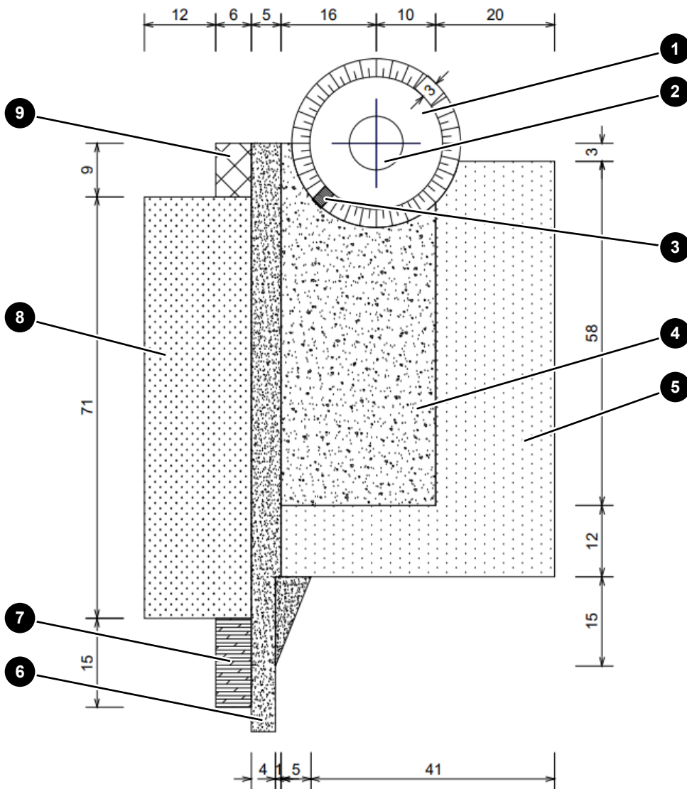
Abb. 14: Alternativer Arbeitsbereich am WEA-Standort, Baumaß (alle Maßangaben in Meter)
