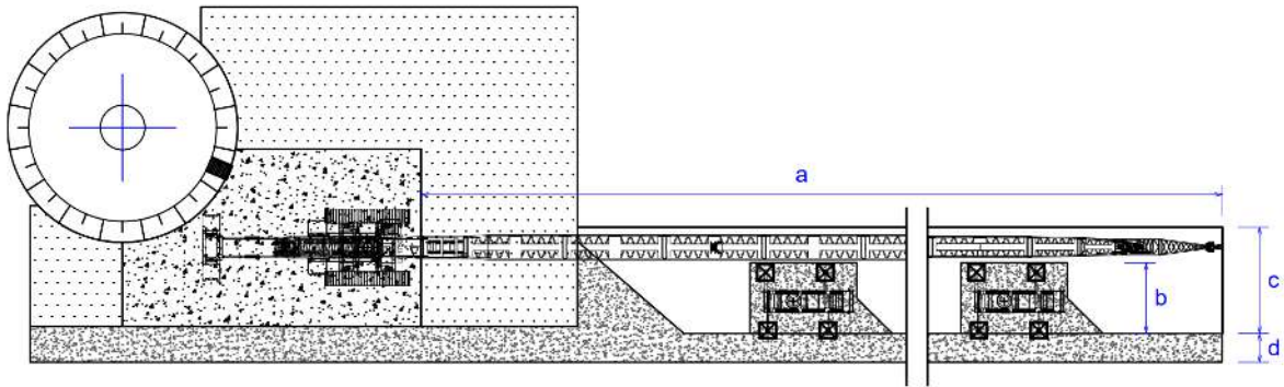
Abb. 13: Kranauslegermontagefläche
