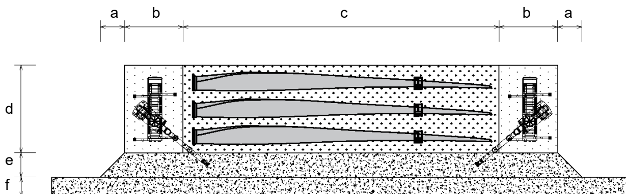
Abb. 16: Rotorblattlagerfläche (Konstruktionsschema)
