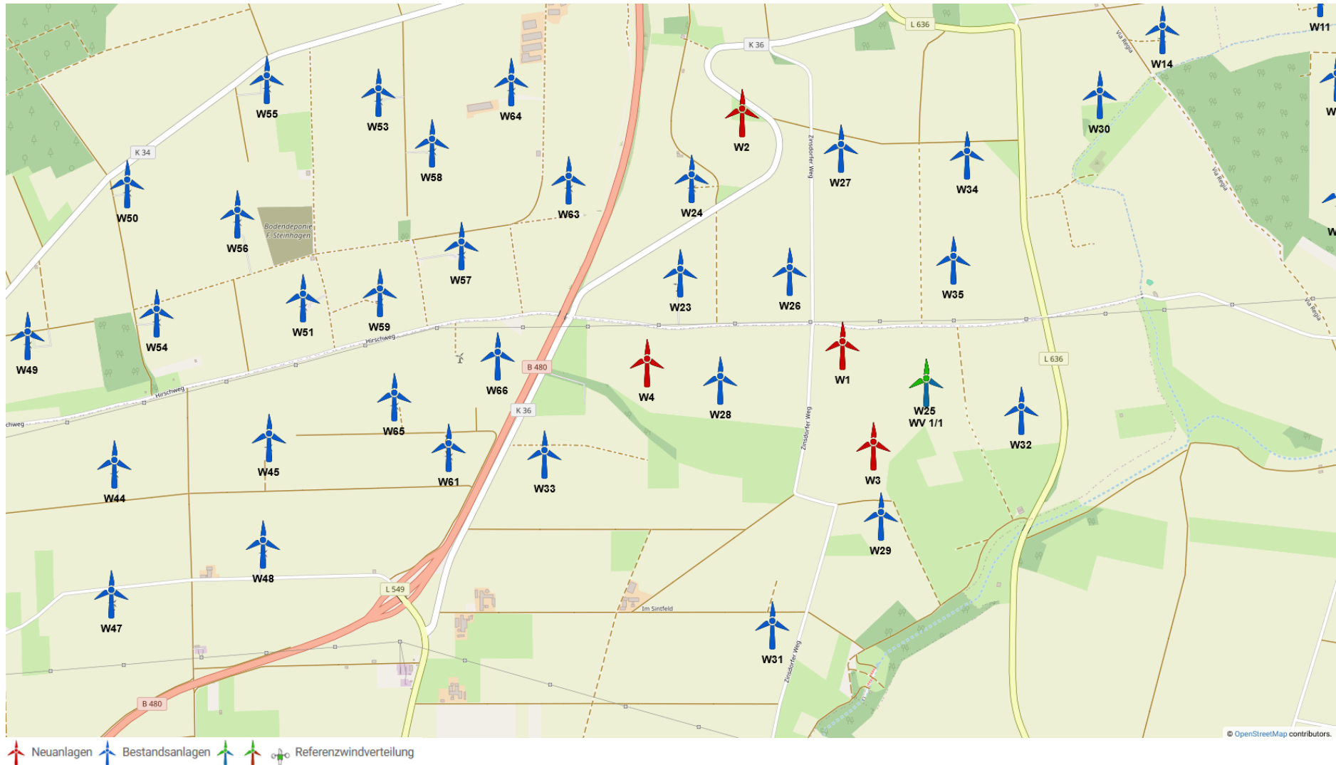
Abbildung 2.2: Zu untersuchende Windparkkonfiguration - Detail; Kartenmaterial: [19.1, 19.2]
