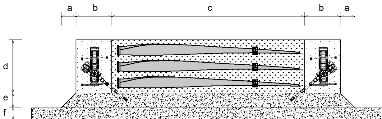
Abb. 13: Rotorblattlagerfläche (Konstruktionschema)
