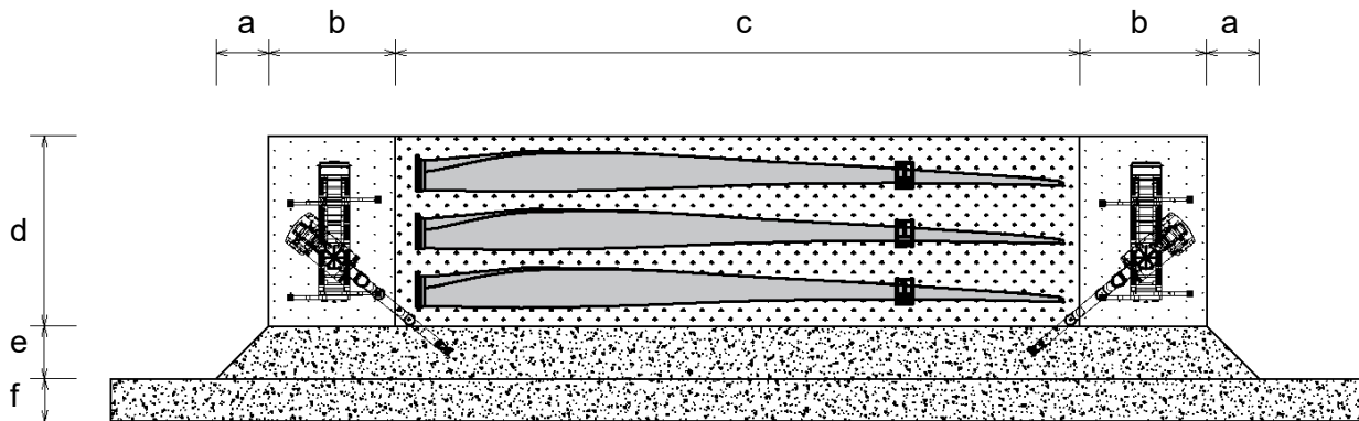
Abb. 14: Rotorblattlagerfläche (Konstruktionschema)
