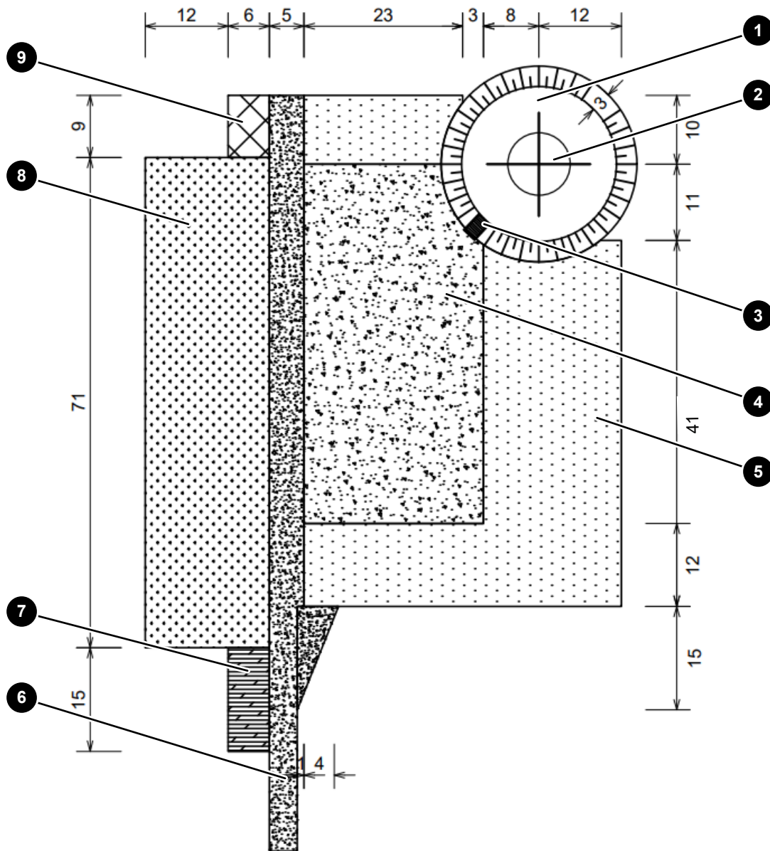
Abb. 10: Arbeitsbereich am WEA-Standort, Baumaß (alle Maßangaben in Meter)
