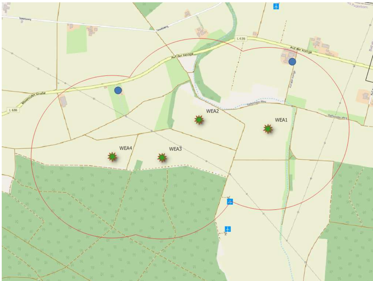
Abbildung 5: geplante WEA mit Radius (rote Linie) jeweils 3-fache Gesamtanlagenhöhe und nahegelegene Wohnbebauungen (blaue Markierungen); Quelle: Google Satellite (durch Verfasser ergänzt)
