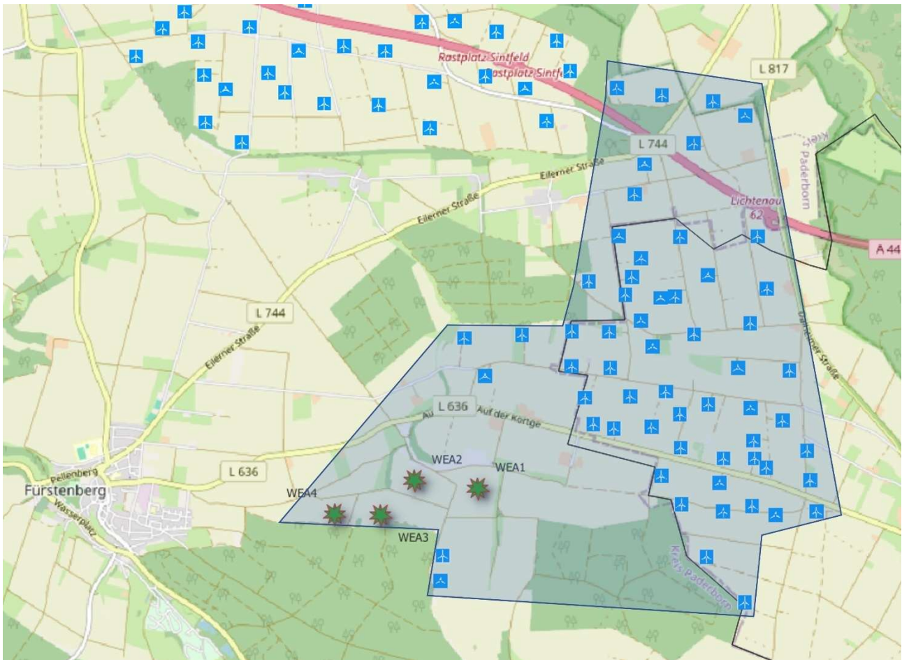
Abbildung 4 Abgrenzung des Untersuchungsgebietes der Windfarm „Fürstenberg“ (blau) mit geplanten Standorten der vier geplanten WEA (grüne Sterne) (nicht maßstäblich)
