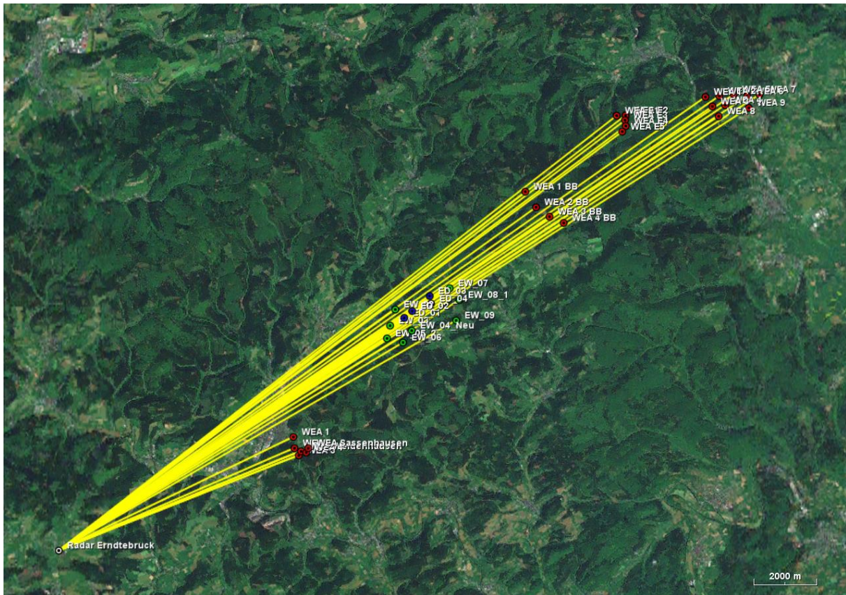
Abbildung 2: Luftaufnahme des Windparks Ohrenbach mit den geplanten Windenergieanlagen (grün), den genehmigten jedoch nicht gebauten da beklagten WEA (blau) sowie der relevanten Vorbelastung (rot). Die Einstrahlungsrichtungen bzgl. der Radaranlage Erndtebrück sind gelb dargestellt. Um eine bessere Übersicht zu gewährleisten wurden die Bezeichnungen von einzelnen Anlagen teilweise ausgeblendet.
