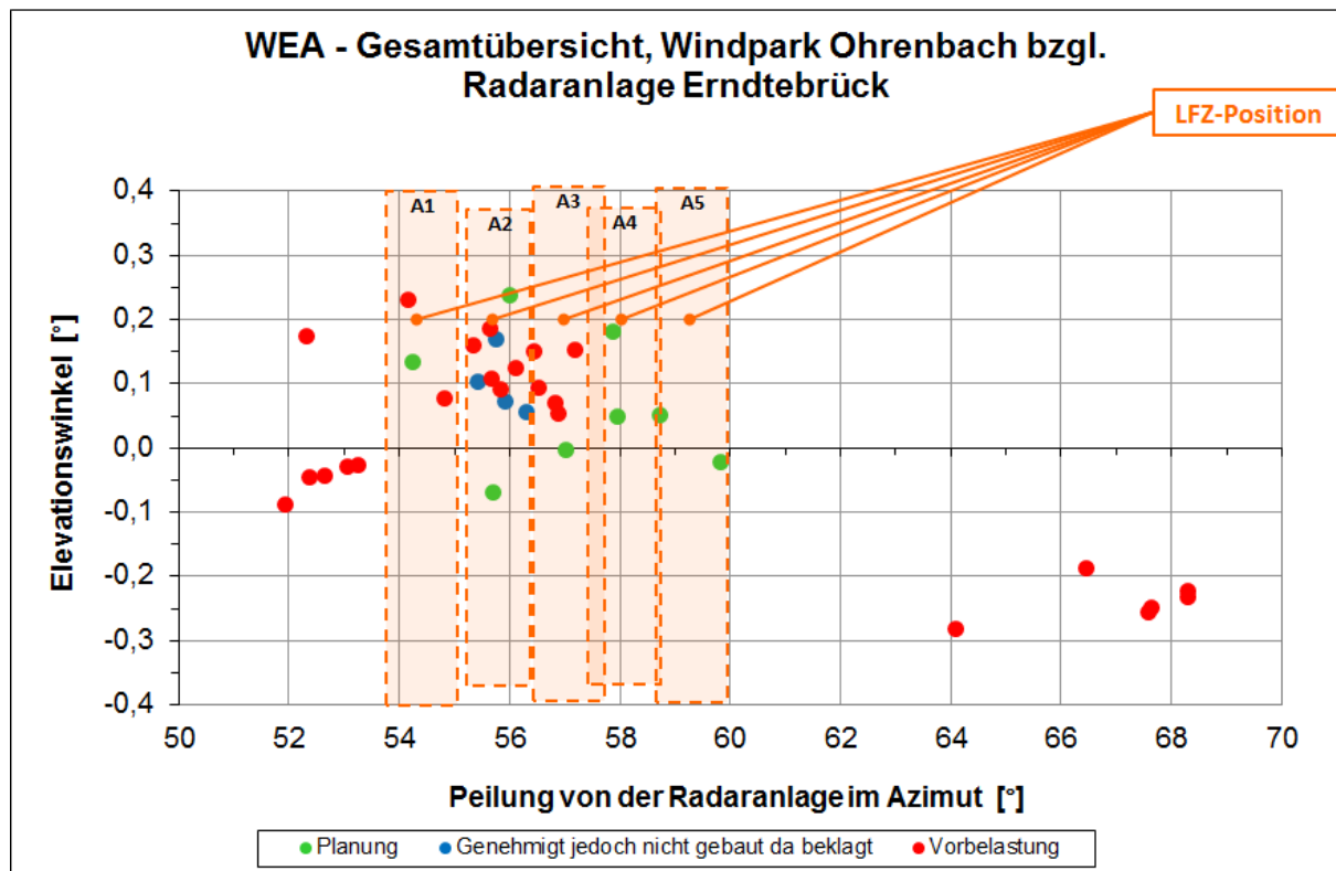
Abbildung 12: Perspektive zur Gondelanordnung gemäß Azimut und Elevation für die Position des Radars Erndtebrück. Die Bereiche der analysierten Teilanordnungen sind durch farbige Flächen gekennzeichnet. Die Richtung und Elevation des angenommenen Lfz ist dargestellt.
