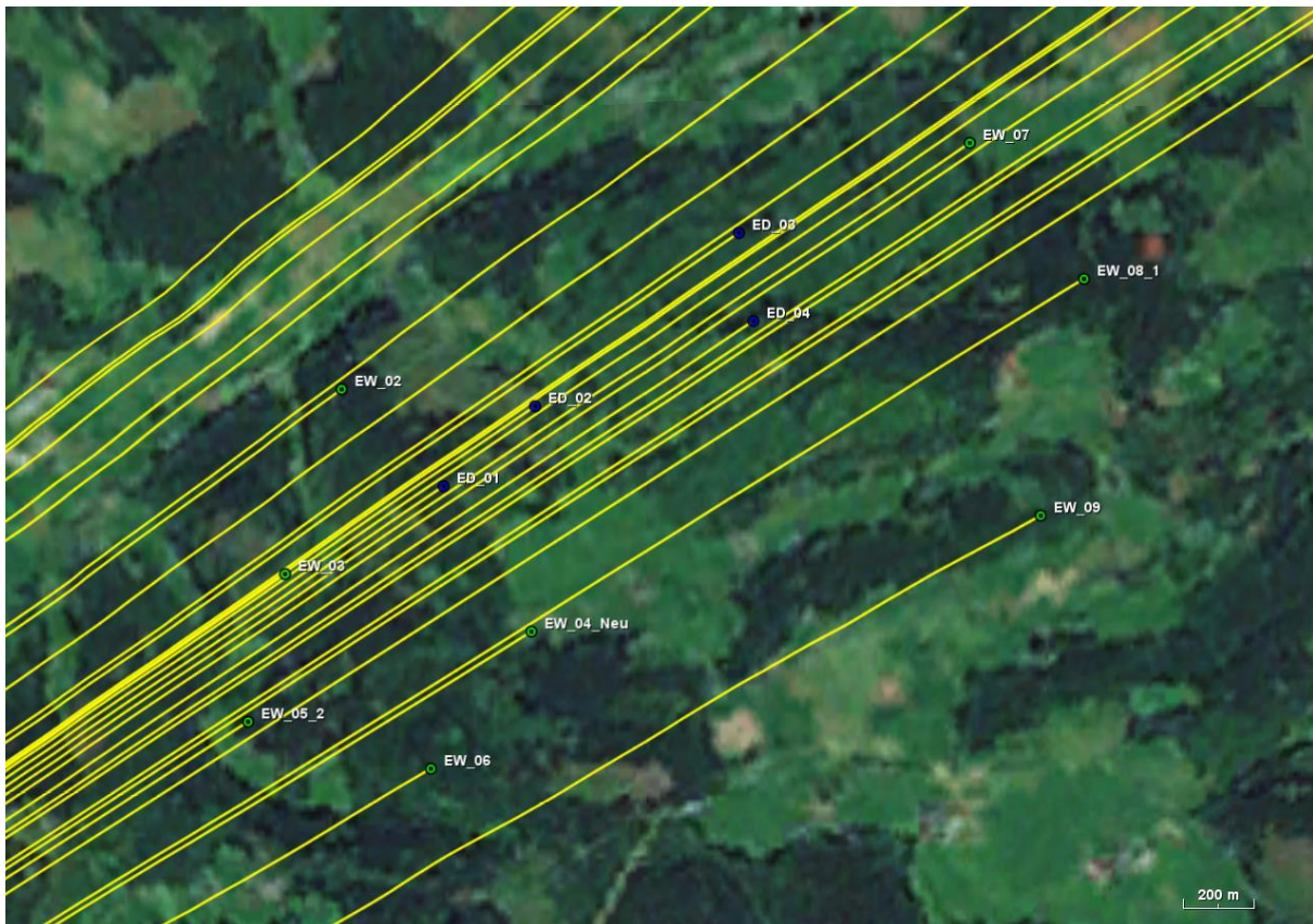
Abbildung 13: Übersicht über den Windpark Ohrenbach mit den geplanten Windenergieanlagen (grün), den genehmigten jedoch nicht gebauten da beklagten WEA (blau) sowie der relevanten Vorbelastung (rot). Die Einstrahlungsrichtungen bzgl. der Radaranlage Erndtebrück sind gelb dargestellt.
