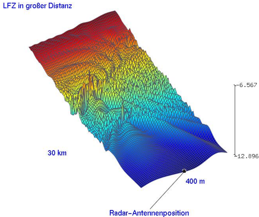
Abbildung 6: Reflexions- und Streufeldausbildung für die Anordnung A1 im Einflussbereich der Radaranlage Erndtebrück
