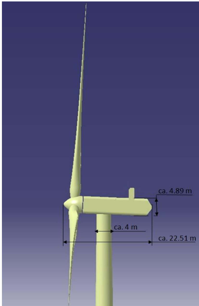
Abbildung 1: Schematische Objektgeometrie für die geplante WEA-Bauform Vestas V162 mit ca. 162 m Rotor
