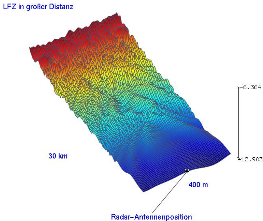
Abbildung 8: Reflexions- und Streufeldausbildung für die Anordnung A3 im Einflussbereich der Radaranlage Erndtebrück
