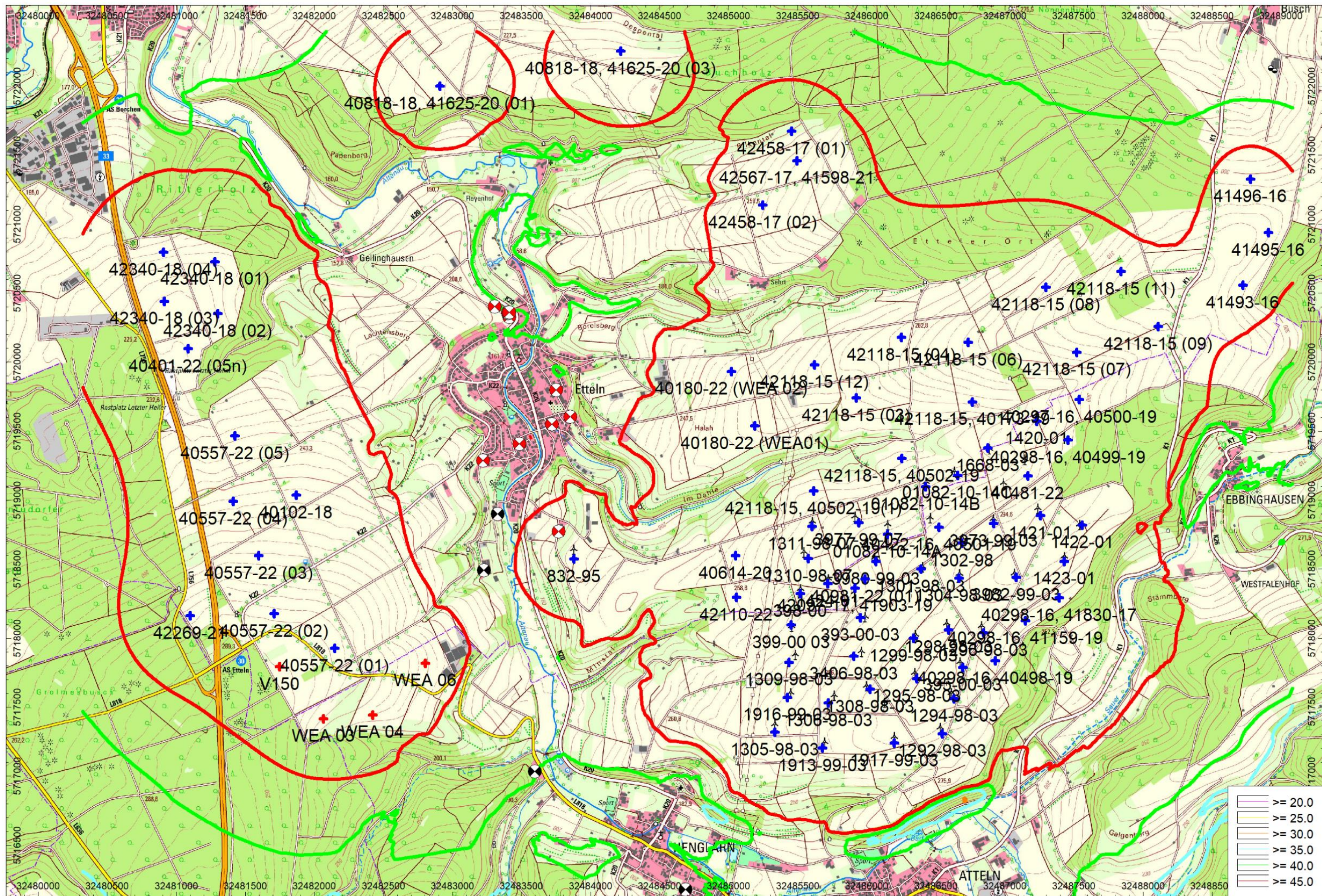
Abbildung 17 Schallausbreitungskarte Gesamtbelastung
