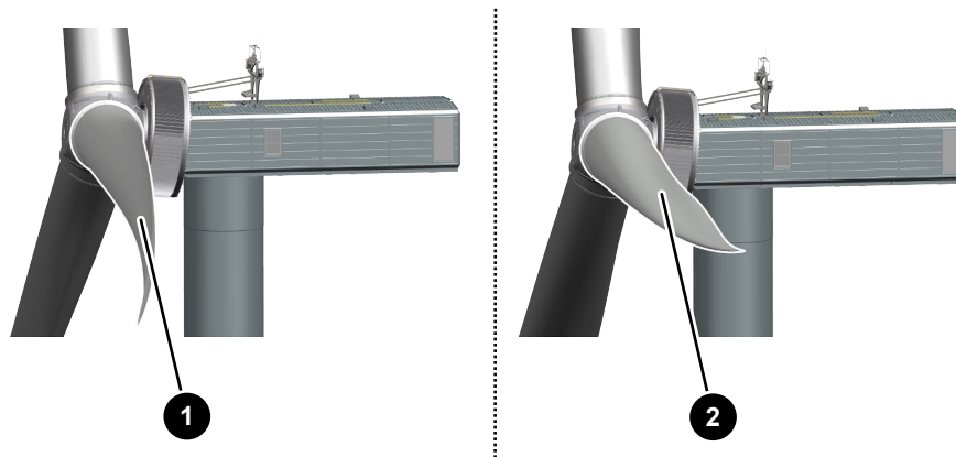
Abb. 3: Besondere Rotorblattstellungen
