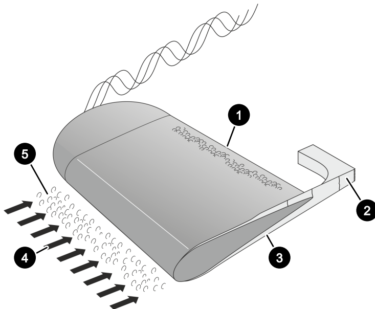
Abb. 1: Strömung am Rotorblatt
