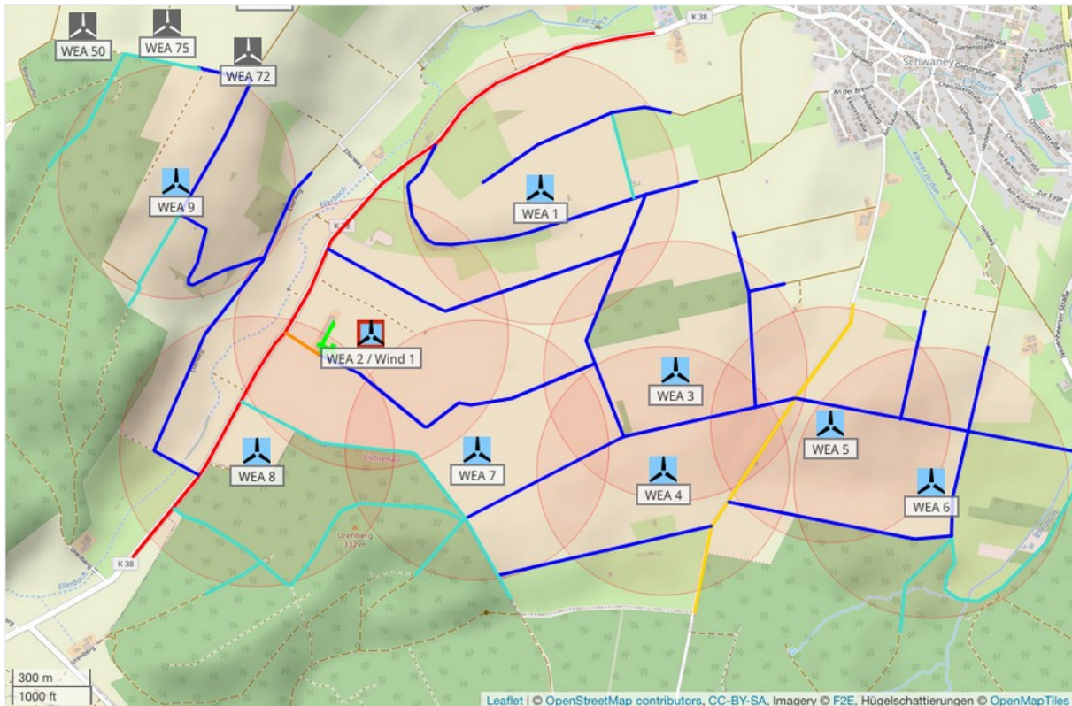
Abbildung 4.3.1: Potentielle Gefährdungsbereiche der WEA und Schutzobjekte am Standort Schwaney Süd (Karte /1.4/).
