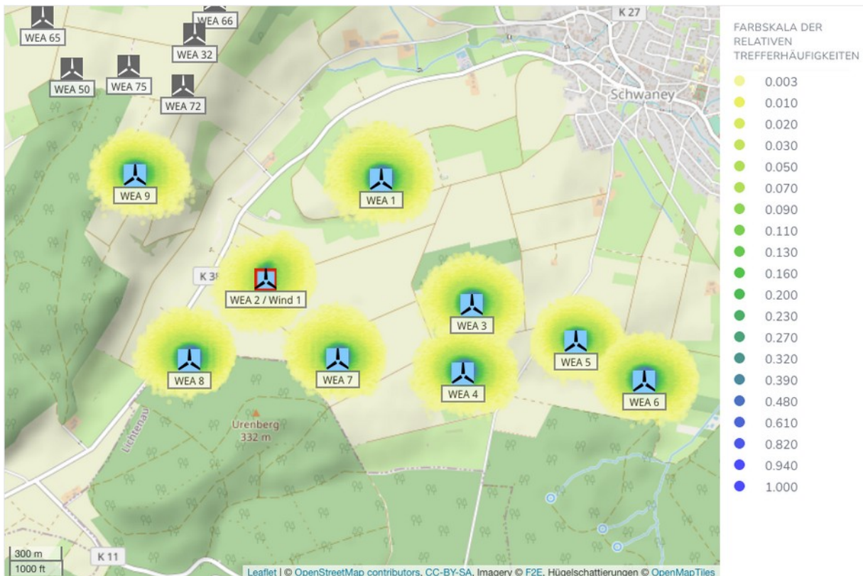
Abbildung A.1.1: Trefferhäufigkeiten von Eisstücken pro Rasterfläche (16m 2 ) und Jahr in der Umgebung der WEA 1 - 9 am Standort Schwaney Süd für eine Azimut-Position nach Abschaltung durch die Eiserkennung für die WEA 2 von 80° (Karte /1.4/).
