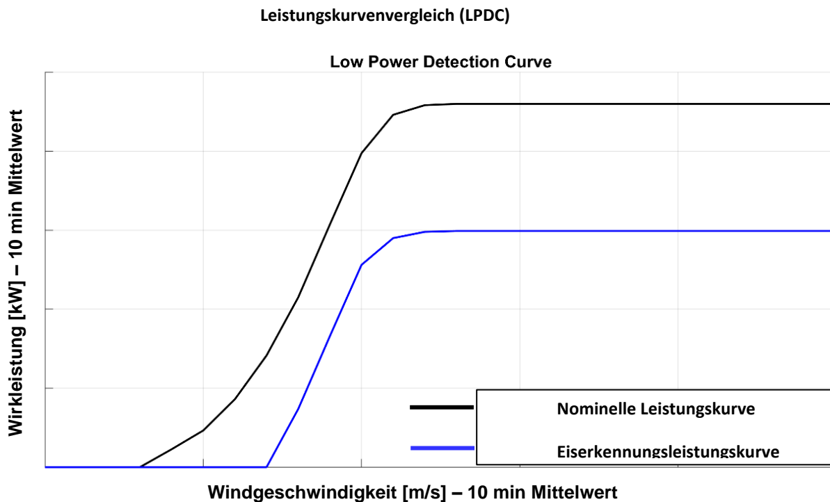
Abbildung 2: Visualisierung des Leistungskurvenvergleichs zur Eiserkennung
