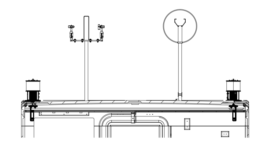
C-C (5:200) Beacon W, rot ES incl. Infrarot / Feuer W, rot ES inkl. Infrarot (100 cd)
