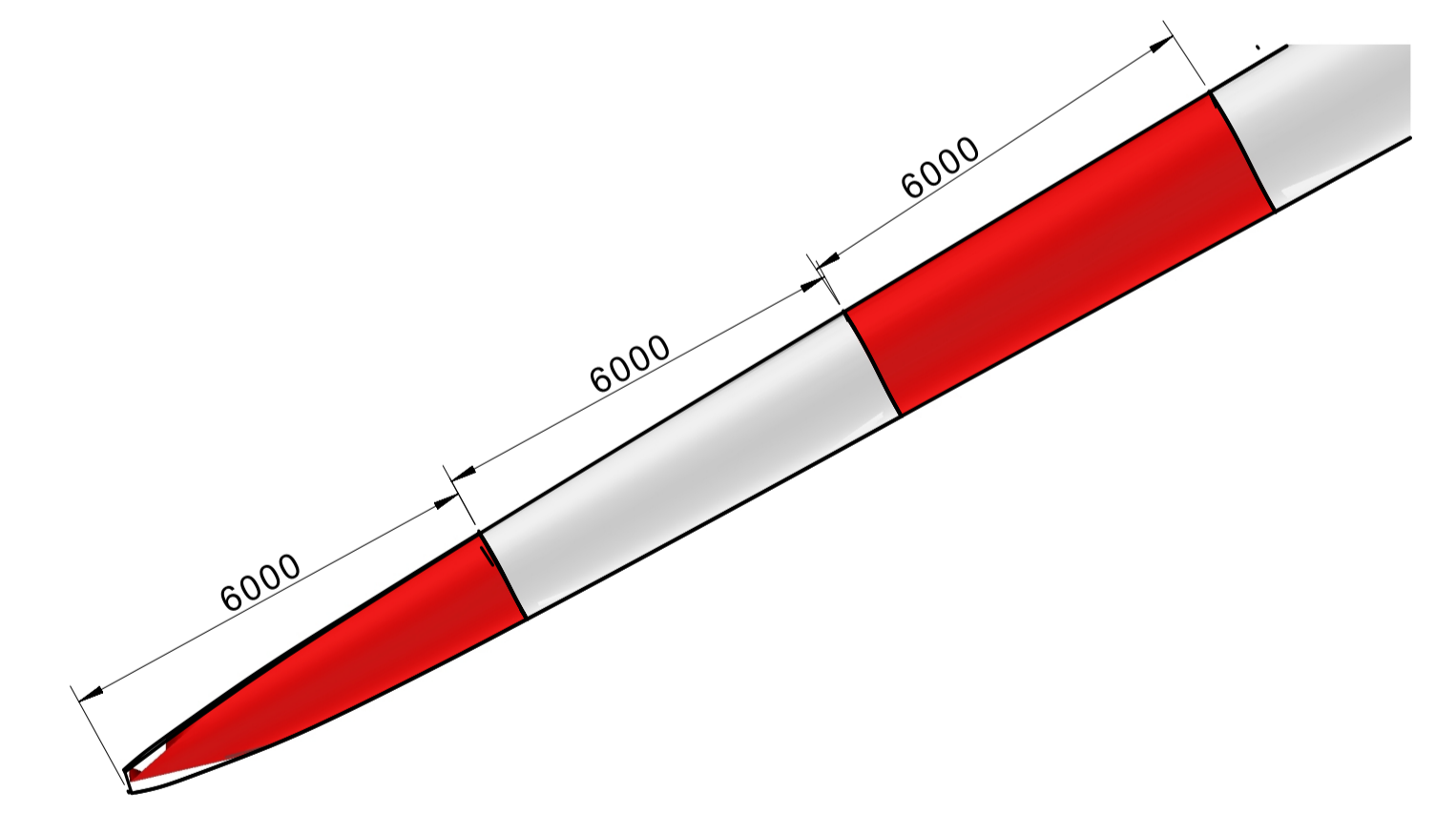
D (1:100) Colour / Farbe: RAL 3020
