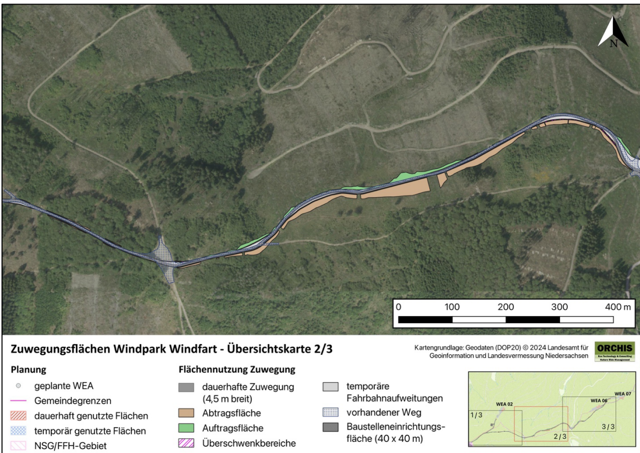
Abbildung 9: Teilabschnitt 2 des Lageplans zur Flächennutzung für die Zuwegung zur Erschließung der geplanten WEA. Eine Darstellung im A3-Format befindet sich im Anhang
