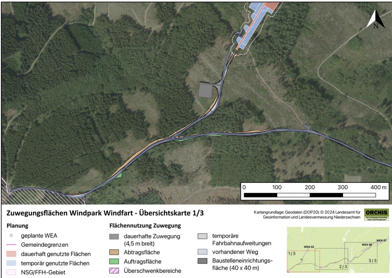
Abbildung 8: Teilabschnitt 1 des Lageplans zur Flächennutzung für die Zuwegung zur Erschließung der geplanten WEA. Eine Darstellung im A3-Format befindet sich im Anhang
