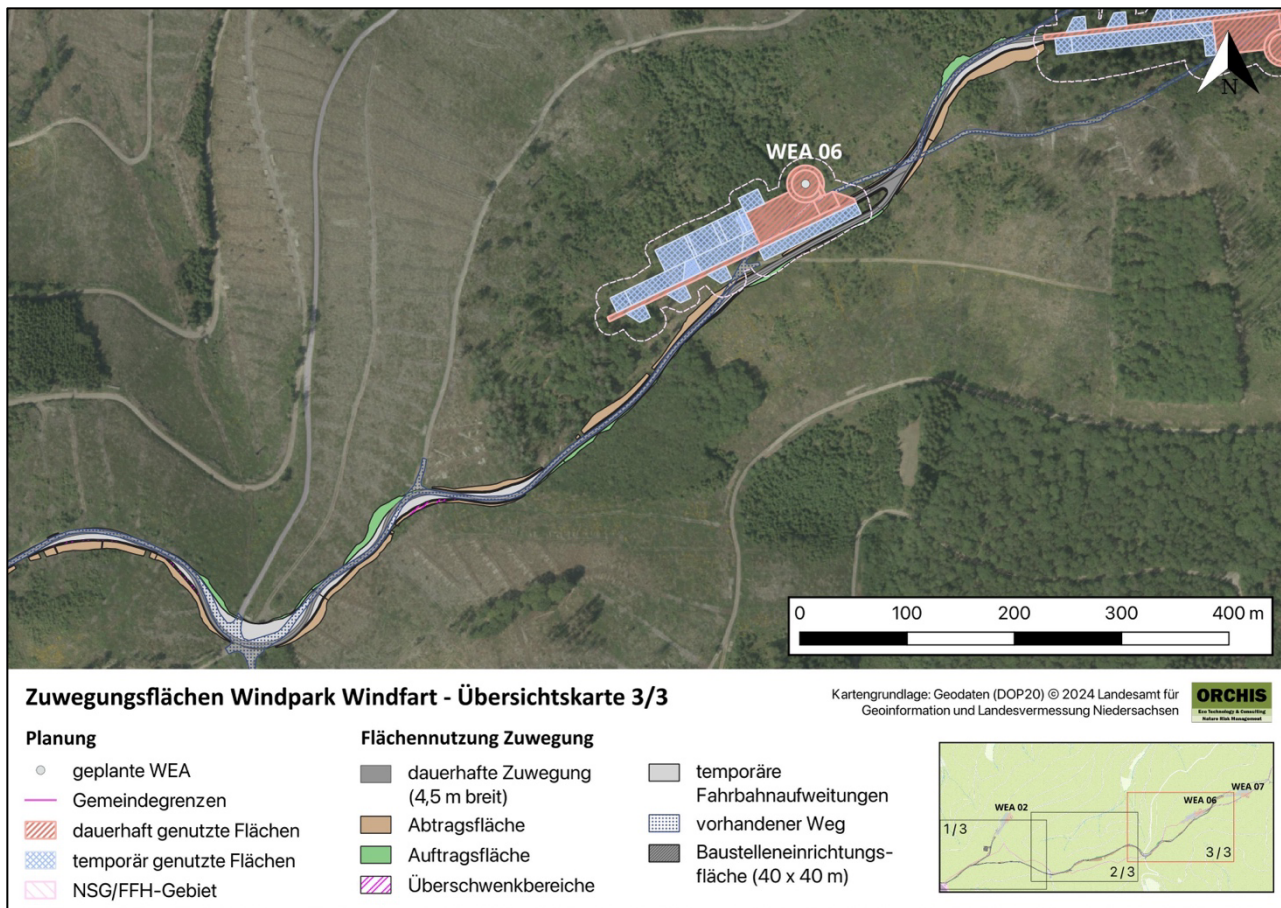
Abbildung 10: Teilabschnitt 3 des Lageplans zur Flächennutzung für die Zuwegung zur Erschließung der geplanten WEA. Eine Darstellung im A3-Format befindet sich im Anhang.
