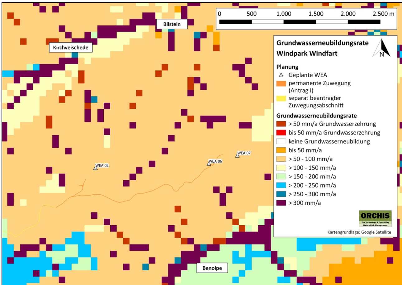
Abbildung 18: Grundwasserneubildungsrate im Bereich der Anlagenstandorte. Quelle: Mittlere jährliche Grundwasserneubildungsrate 1990 – 2020 (berechnet durch FZ Jülich, 2021; LANUV, 2021a))
