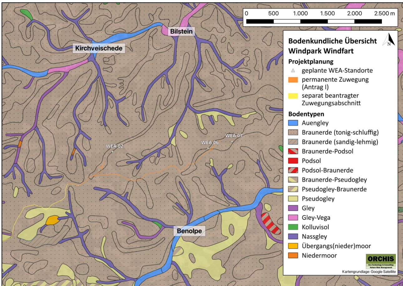
Abbildung 13: Geplante Standorte der WEA im Kontext zur Verbreitung und Vergesellschaftung von Bodenformen. Quelle: BK50 Bodenübersichtskarte (1:50.000) von Nordrhein-Westfalen (GD NRW, 2022)
