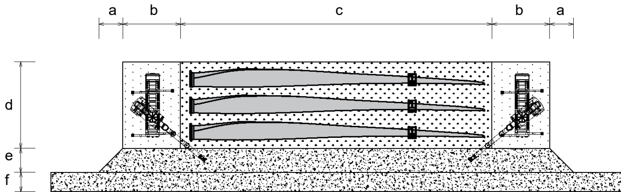
Abb. 14: Rotorblattlagerfläche (Konstruktionsschema)
