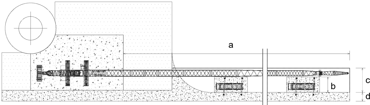
Abb. 13: Kranauslegermontagefläche
