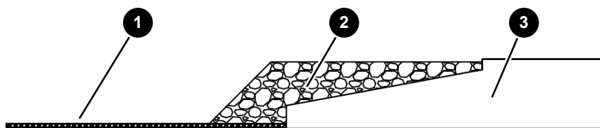
Abb. 10: Fundament auf GOK mit Erdauflast
