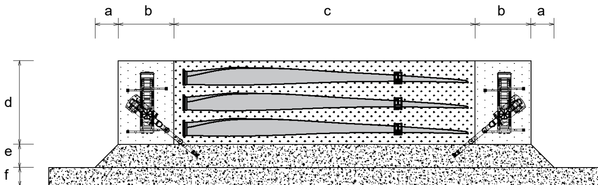
Abb. 13: Rotorblattlagerfläche (Konstruktionsschema)
