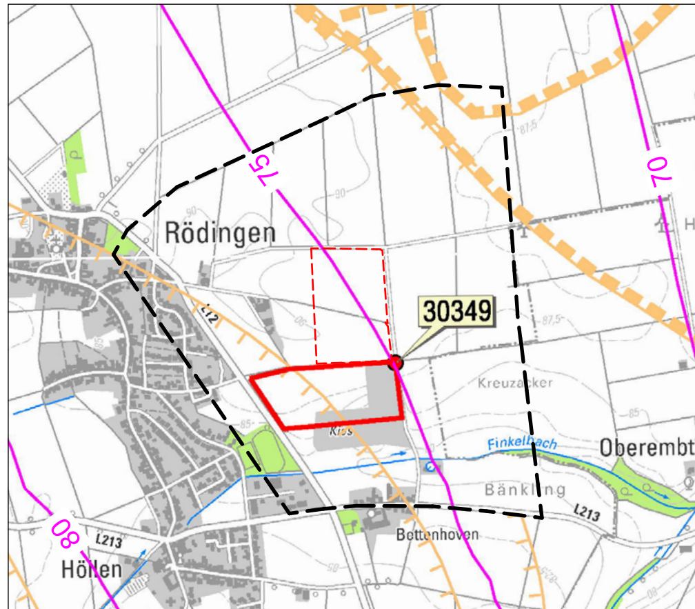
GRUNDWASSERGLEICHEN, ENZZUSTAND 2200
