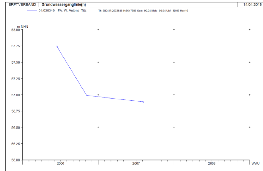
GRUNDWASSERGANGLINIE, MESSSTELLE 30349
