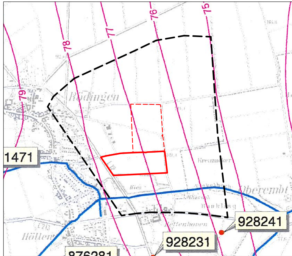
GRUNDWASSERGLEICHEN, OKTOBER 1955
