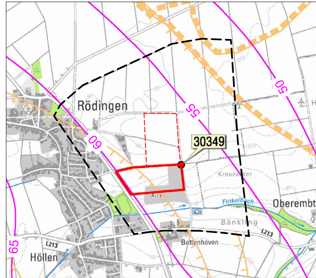
GRUNDWASSERGLEICHEN, OKTOBER 2013
