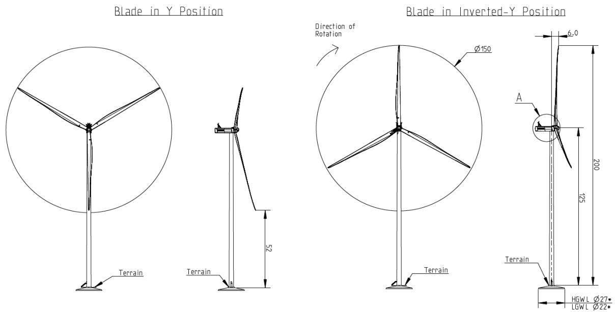
Abbildung 1: Übersichtszeichnung einer Vestas V150-6.0 mit 125 m Nabenhöhe (Quelle: VestasOnline)
