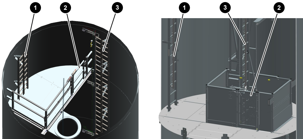
Abb. 8: Ausstiegspodest der Aufstiegshilfe im Stahlturm (links), im Hybridturm (rechts) (Beispiele)
