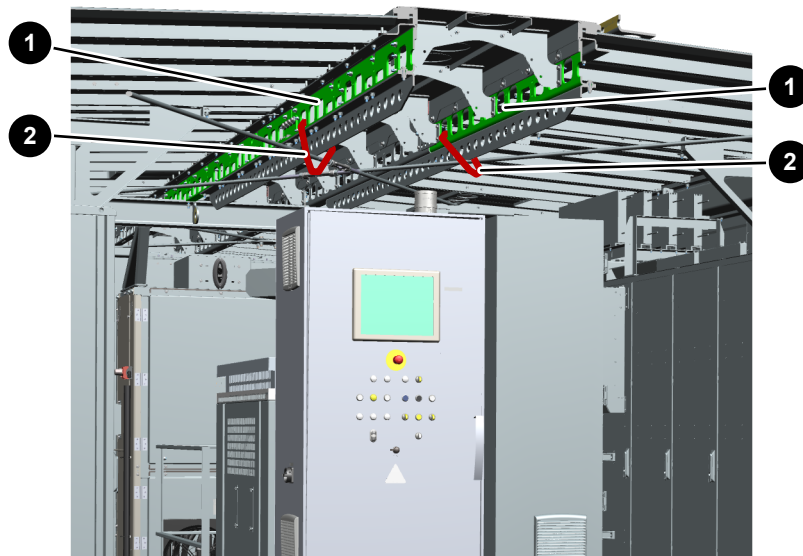
Abb. 3: Befestigungspunkte an den Dachtragschienen (Beispiel)
