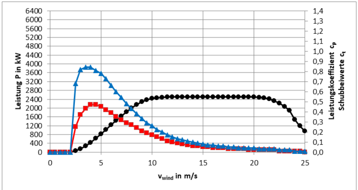
Abb. 1: Leistungs-, c_p - und c_t -Kennlinien E-175 EP5 / 6000 kW Betriebsmodus OM-NR-07-0
