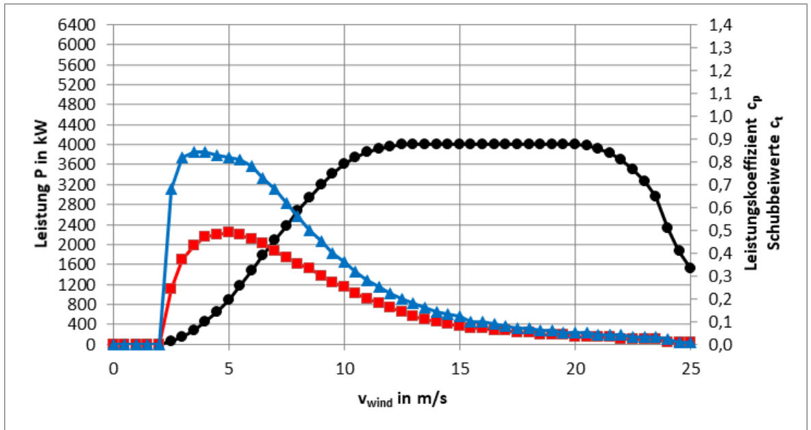
Abb. 1: Leistungs-, c_p - und c_t -Kennlinien E-175 EP5 / 6000 kW Betriebsmodus OM-NR-04-0
