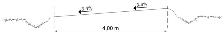
Abb. 8: Seitliches Gefälle
