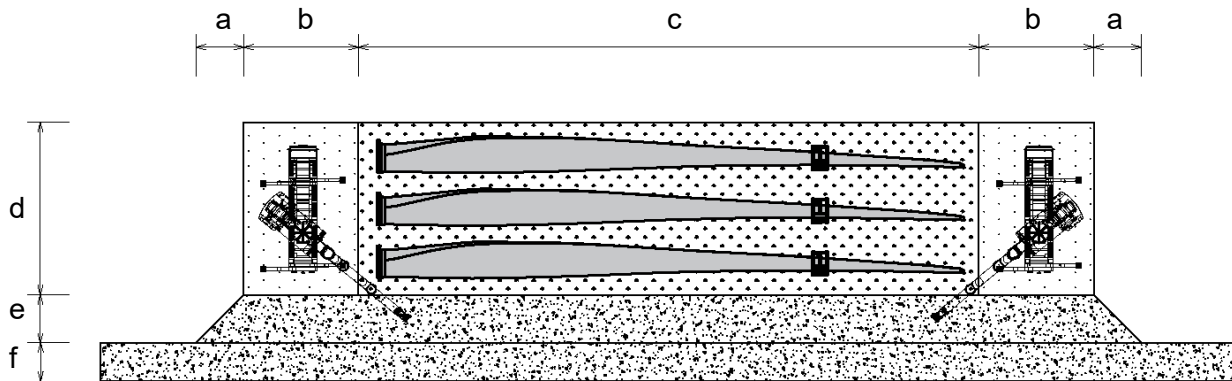
Abb. 16: Rotorblattlagerfläche (Konstruktionsschema)
