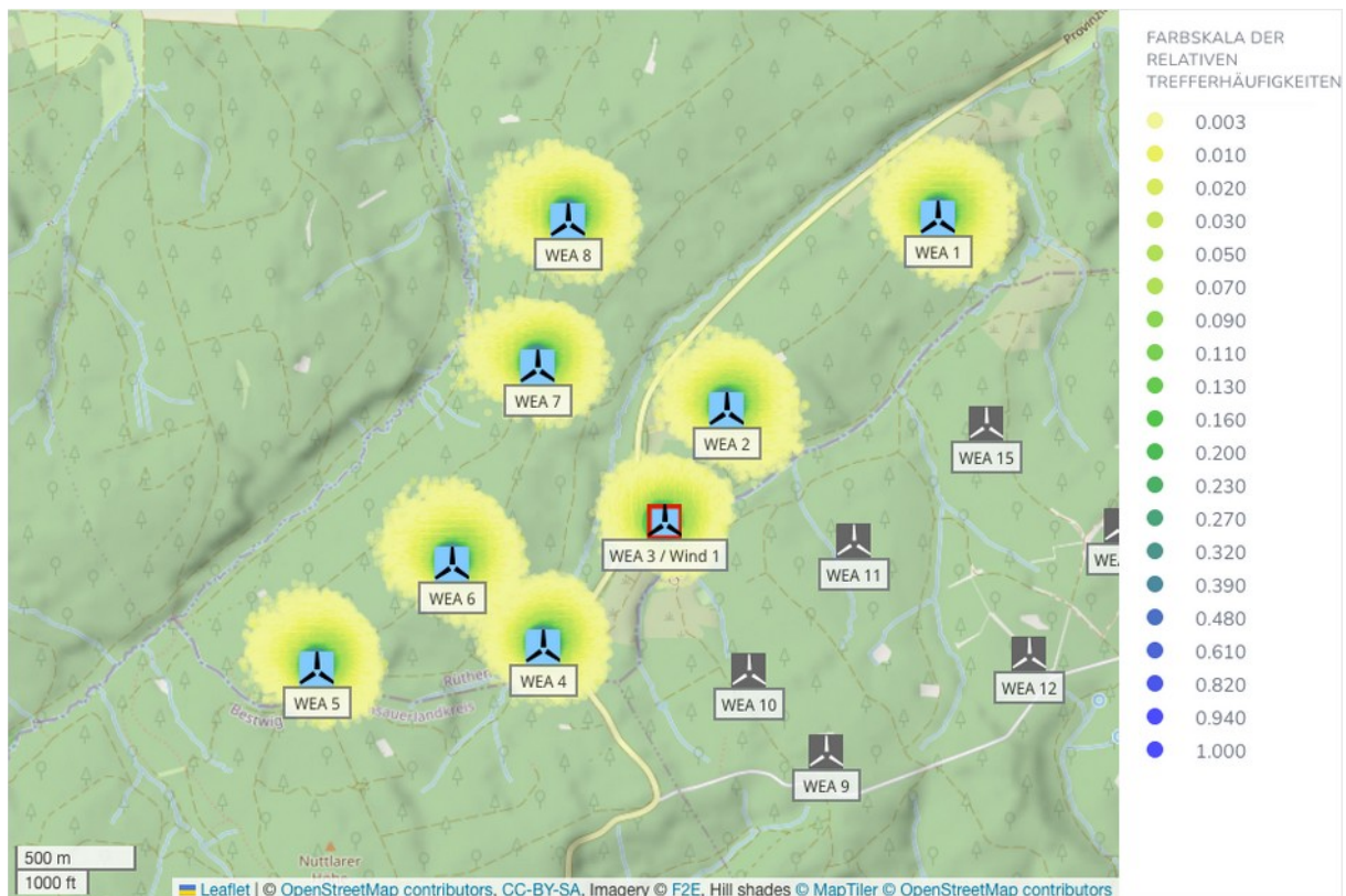
Abbildung A.1.1: Trefferhäufigkeiten von Eisstücken pro Rasterfläche (16m 2 ) und Jahr in der Umgebung der WEA 1 – 8.
