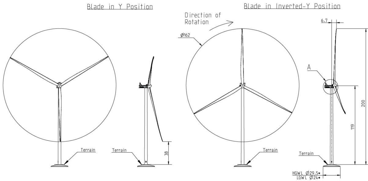
Abbildung 1: Übersichtszeichnung einer Vestas V162-7.2 mit 119 m Nabenhöhe (Quelle: VestasOnline)
